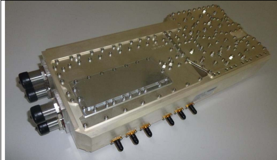
Duplexer
