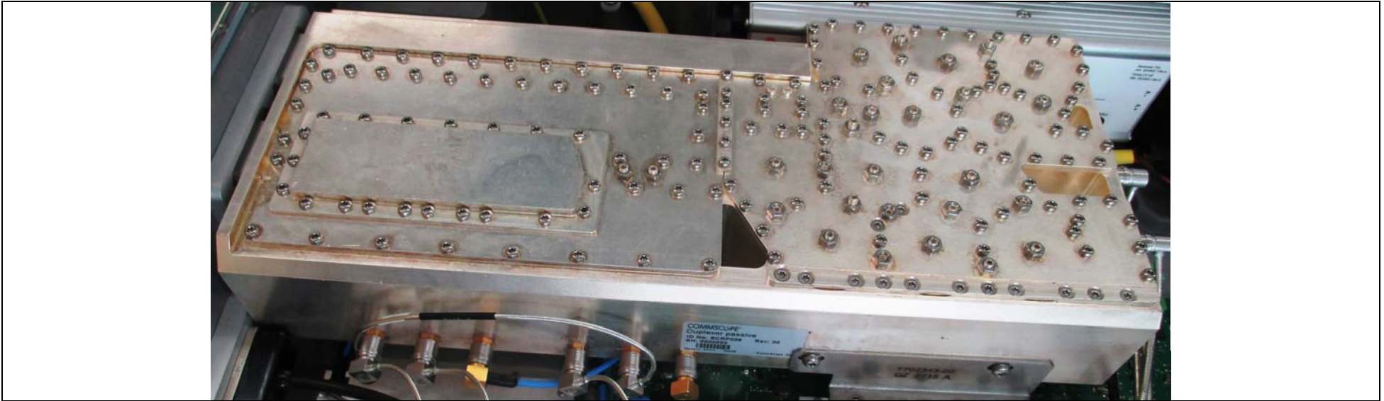
Duplexer
