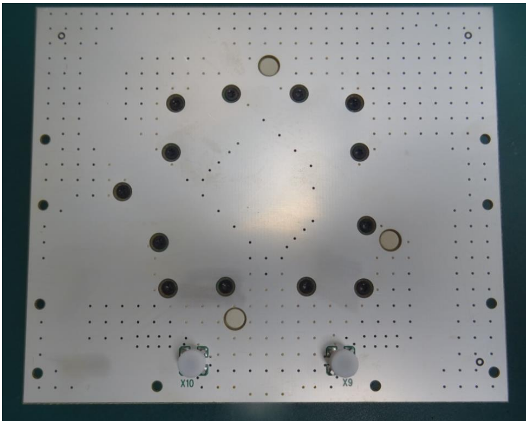
Antenna 7E – 7850491-01 – TOP View
