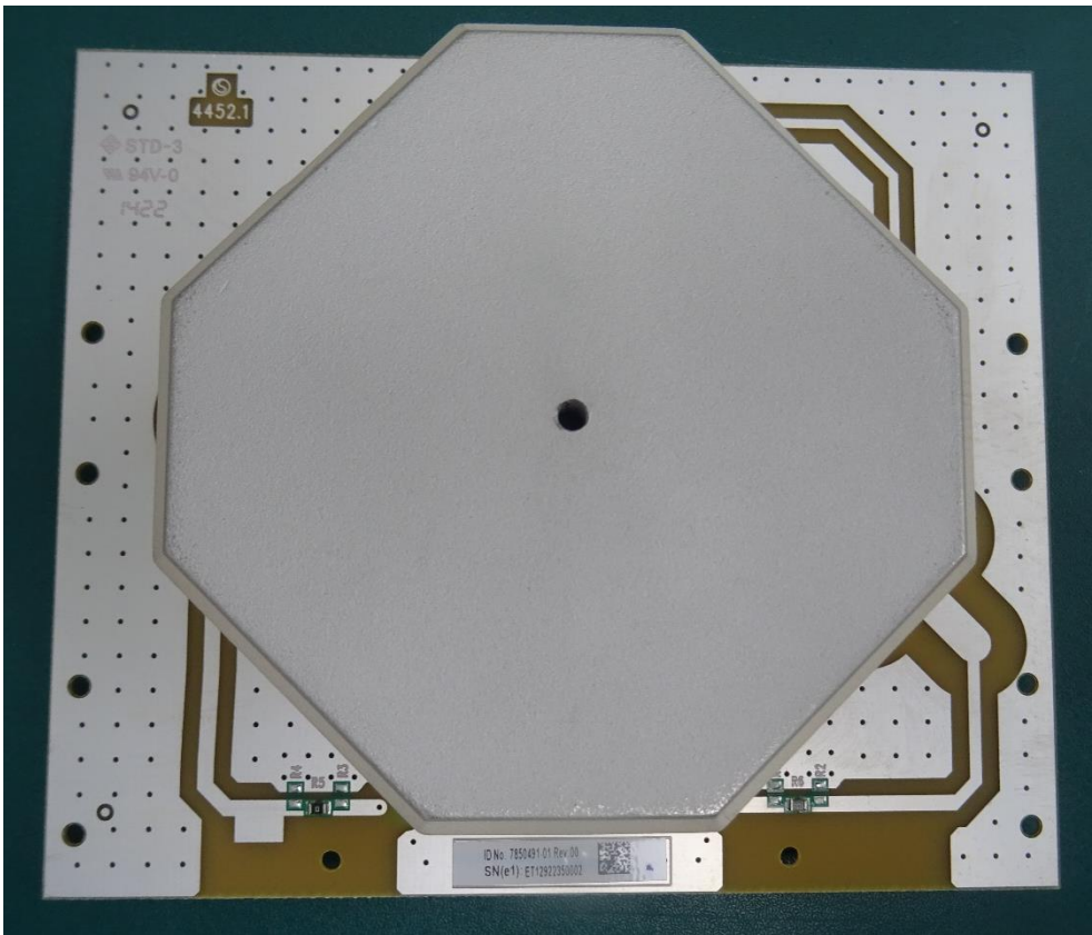
Antenna 7E – 7850491-01 – TOP View
