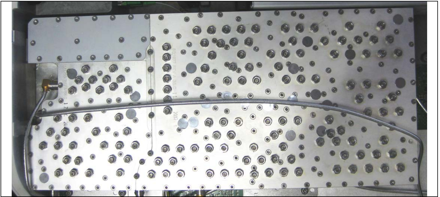
Duplexer
