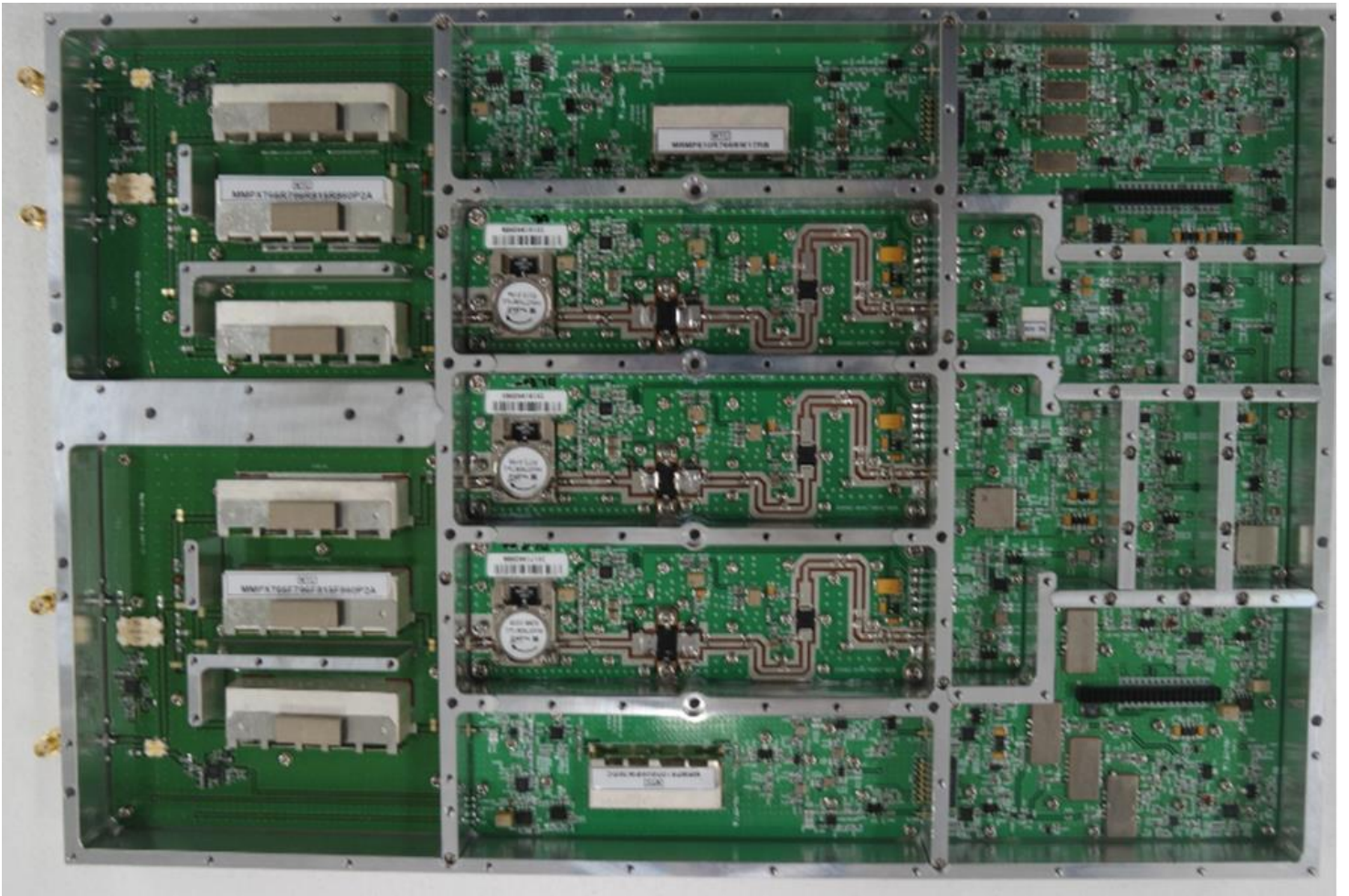
RF Module
