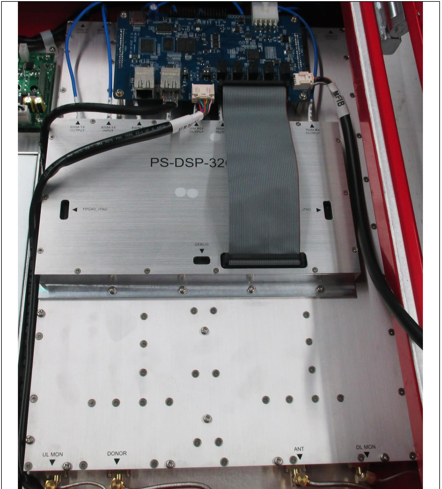
RF-Module
