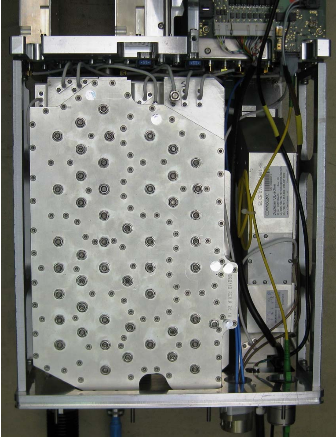
Duplexer
