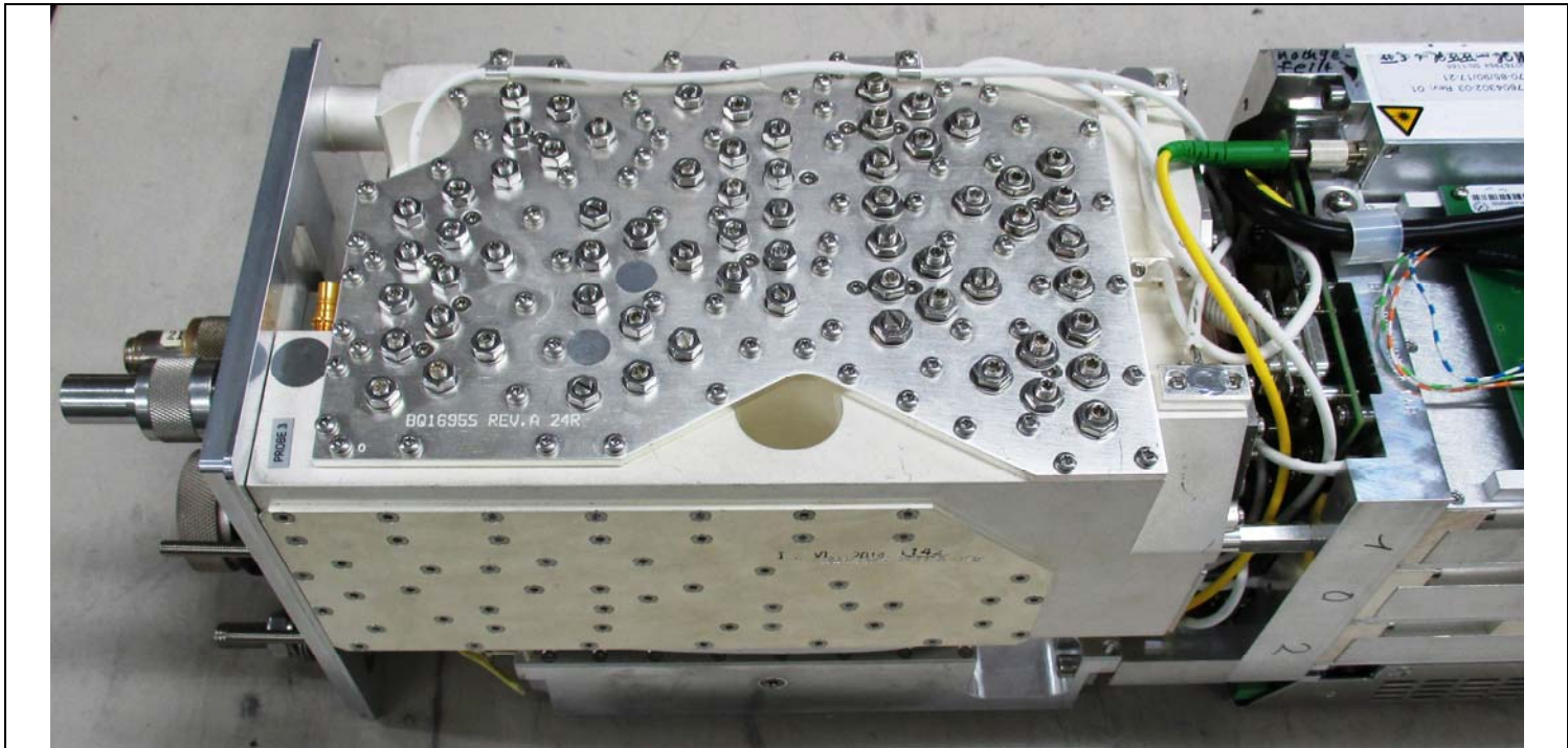
Duplexer
