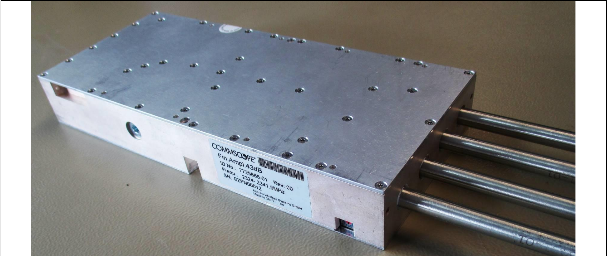
Fin.Ampl.2324-2341.5 43dB 7725865-01
