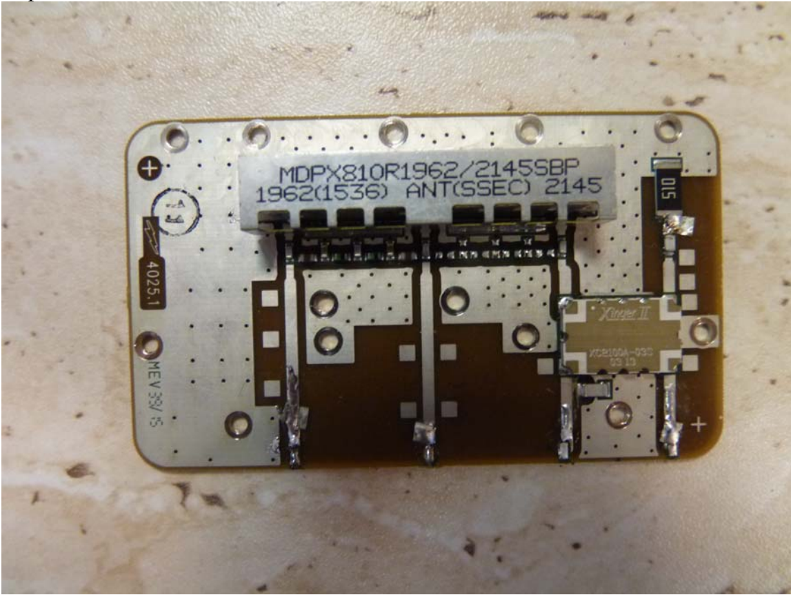
Duplexer PCB 7710715-00
