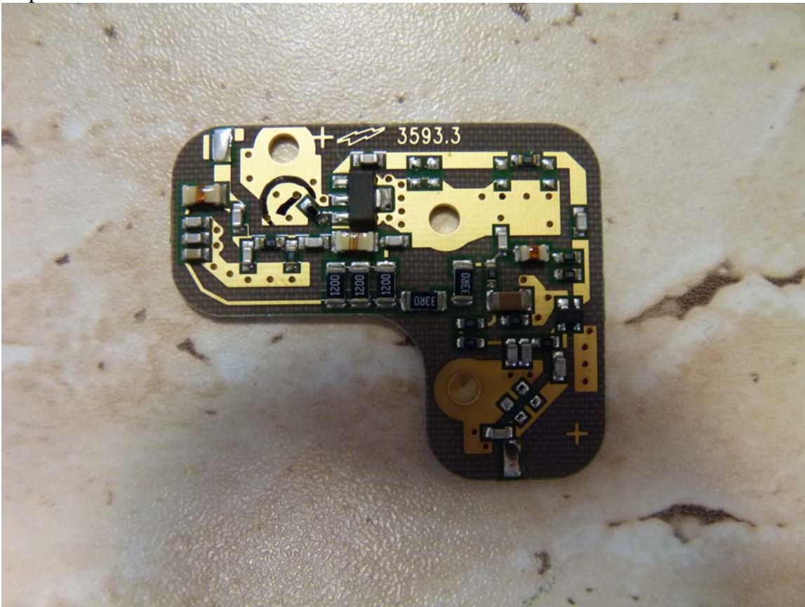
Duplexer PCB 7615458-01
