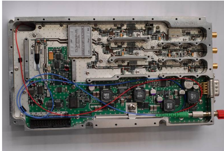
OTRx top:
