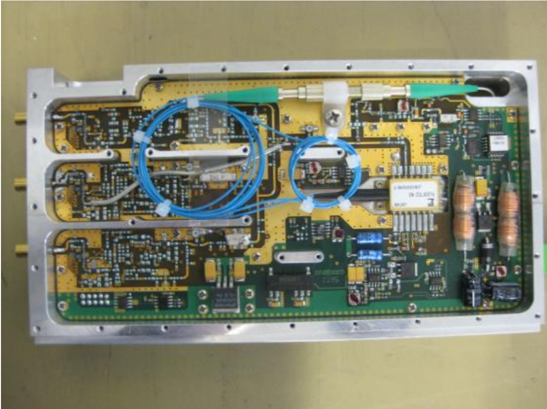
OTRx Bottom
