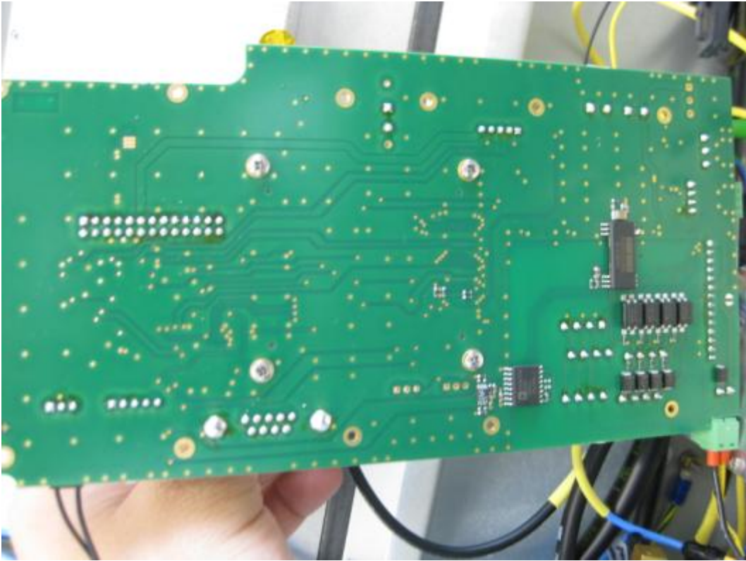
Miniboard Top
