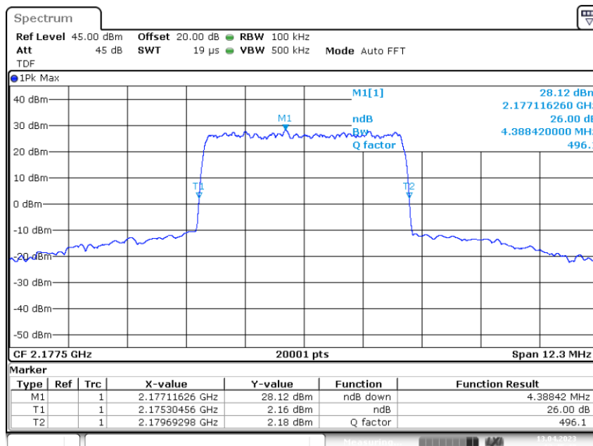
3.4 OCBw AWGN Out +3 2.1775G _26dB
