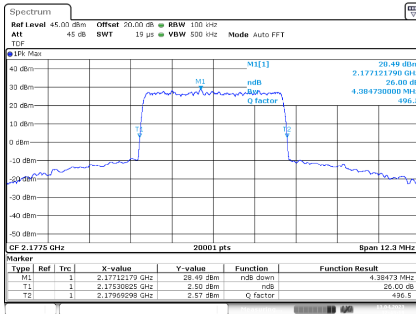
3.4 OCBw AWGN Out -0.3 2.1775G _26dB
