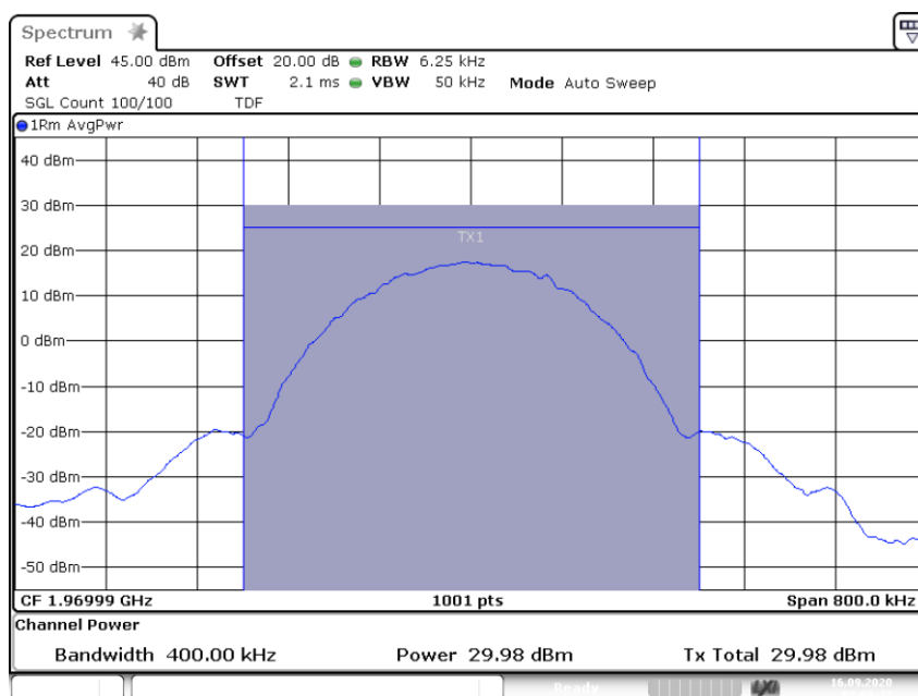
3.5.3 Power GSM Out +3 1.96999G
