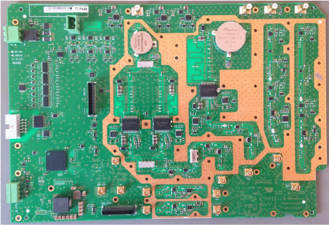
RF1 main 7E/17E – Bottom view
