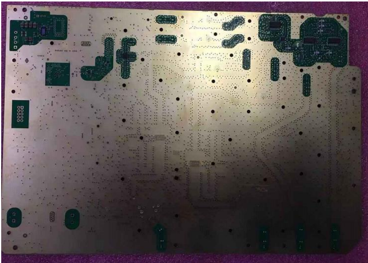
- PCBA 7837503-00 BOT
