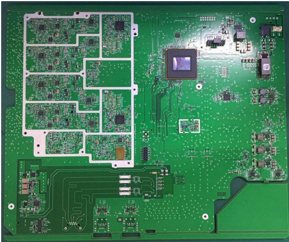
- PCBA 7781249-02 BOT
