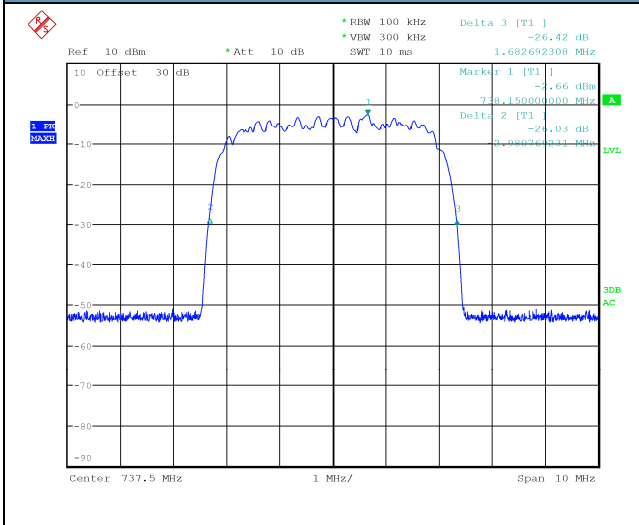
Input
