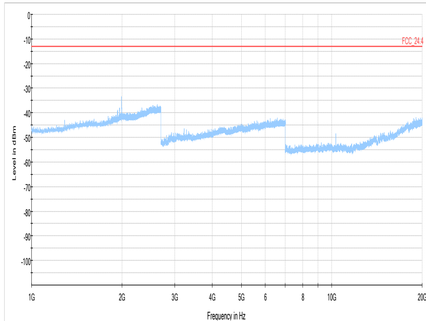
1 GHz - 20 GHz
