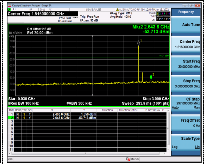
30MHz-3GHz
