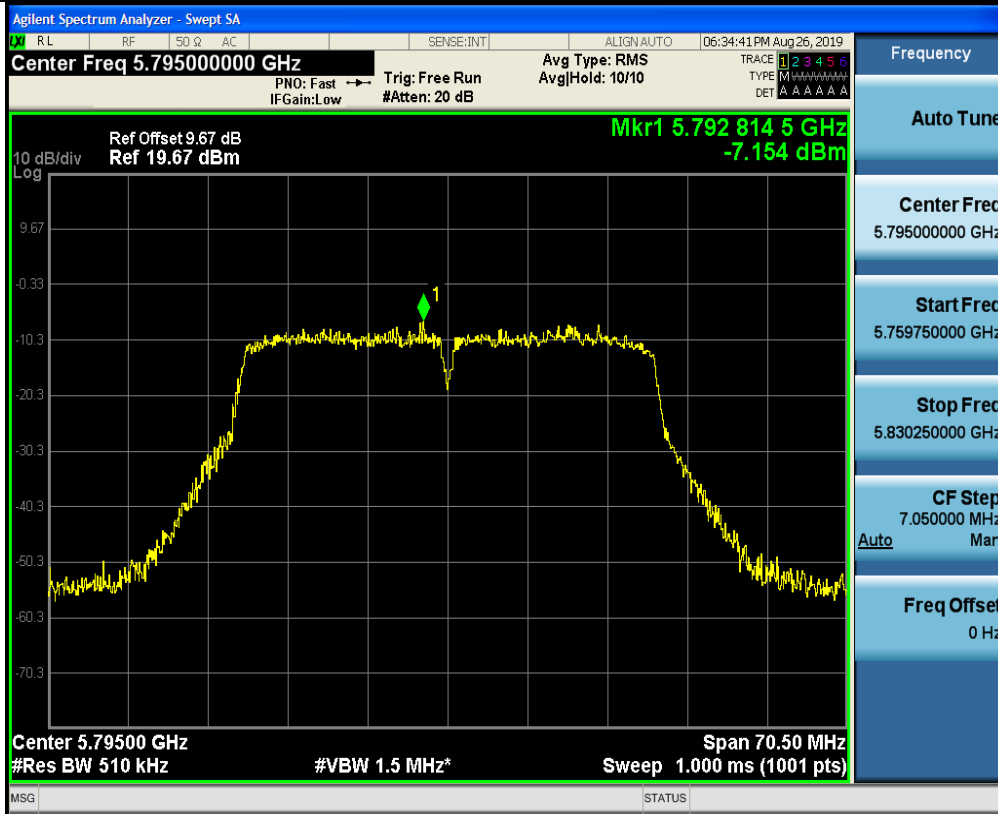
High 802.11ac(HT80)
