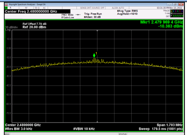
2Mbps / 2480MHz
