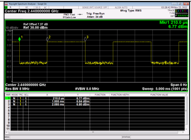
Ton time
