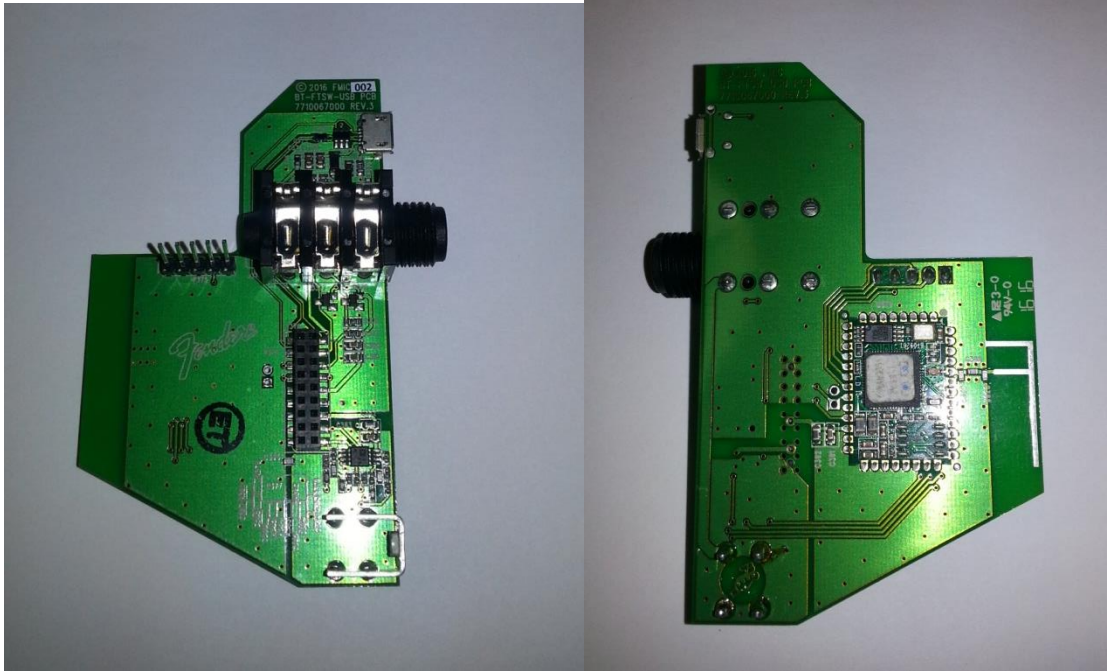
Top Side PCB Module
