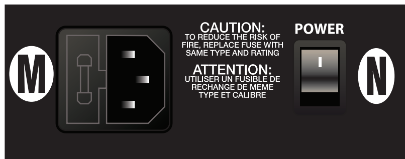
Pannello posteriore del Fighter 10; funzioni e disposizione sono uguali per il Fighter 12.
