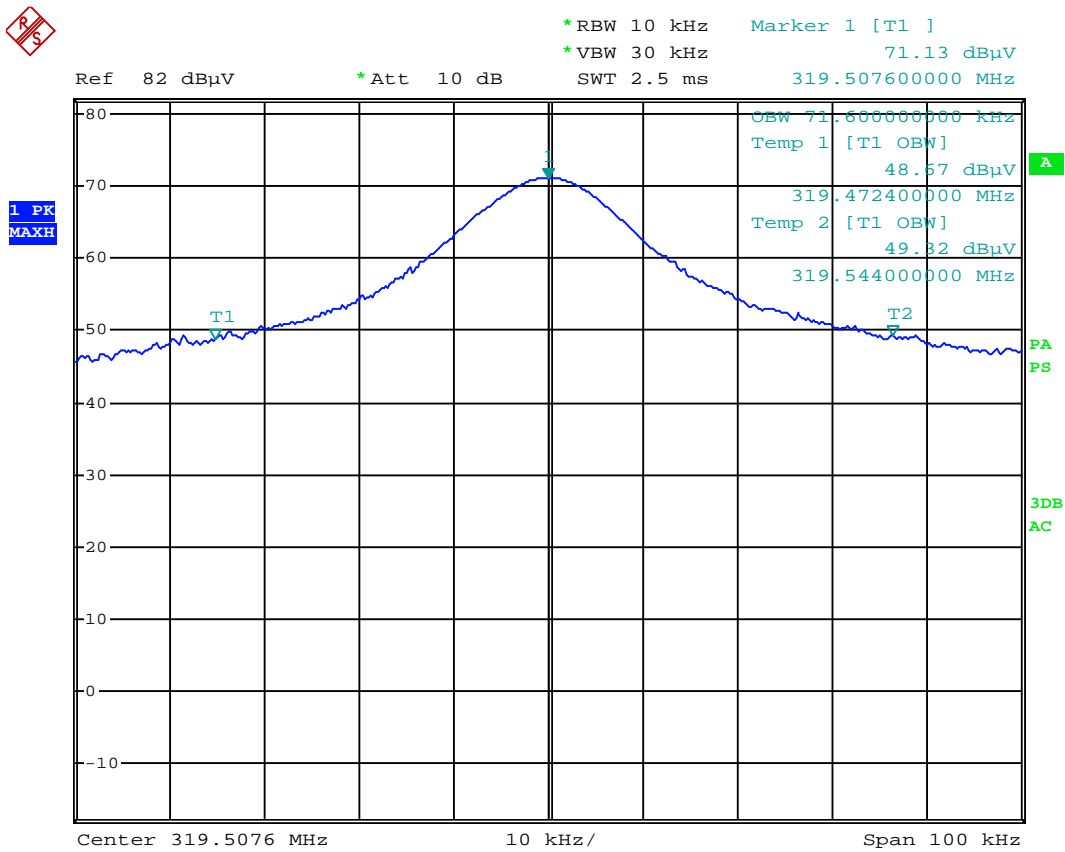
IC 99% OBW
