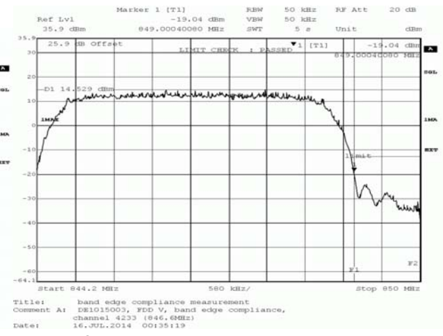
HSUPA FDD5
