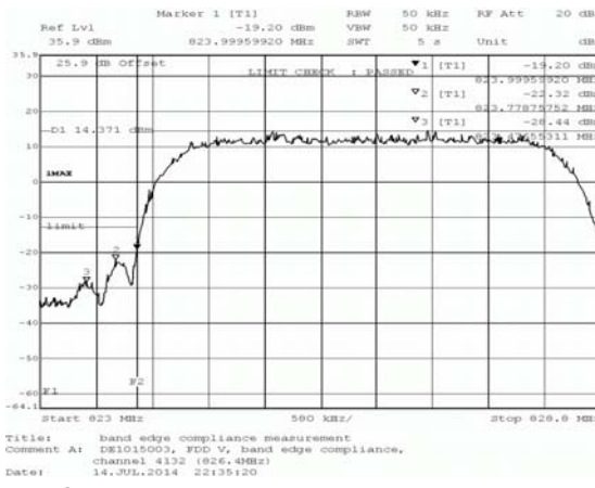
UMTS FDD5
