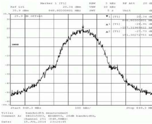
EGDE 850 Band
