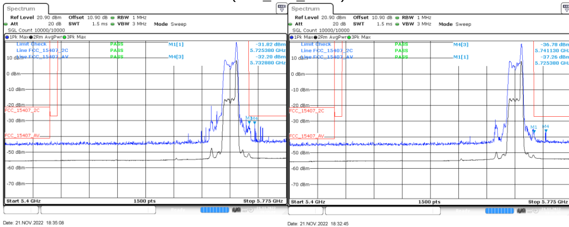
Antenna A
