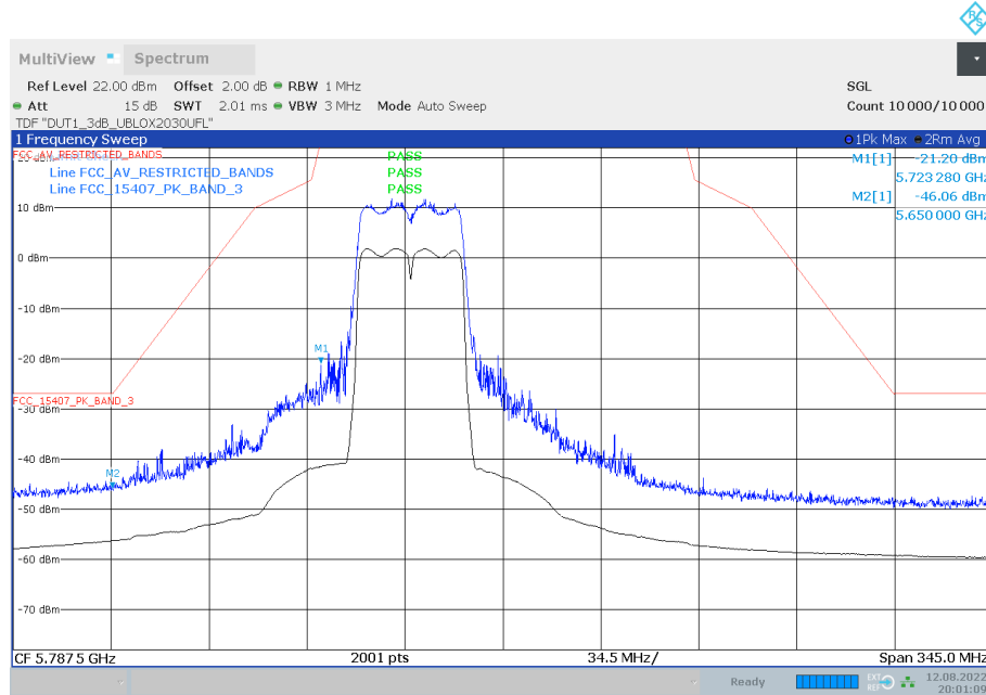
Antenna A
