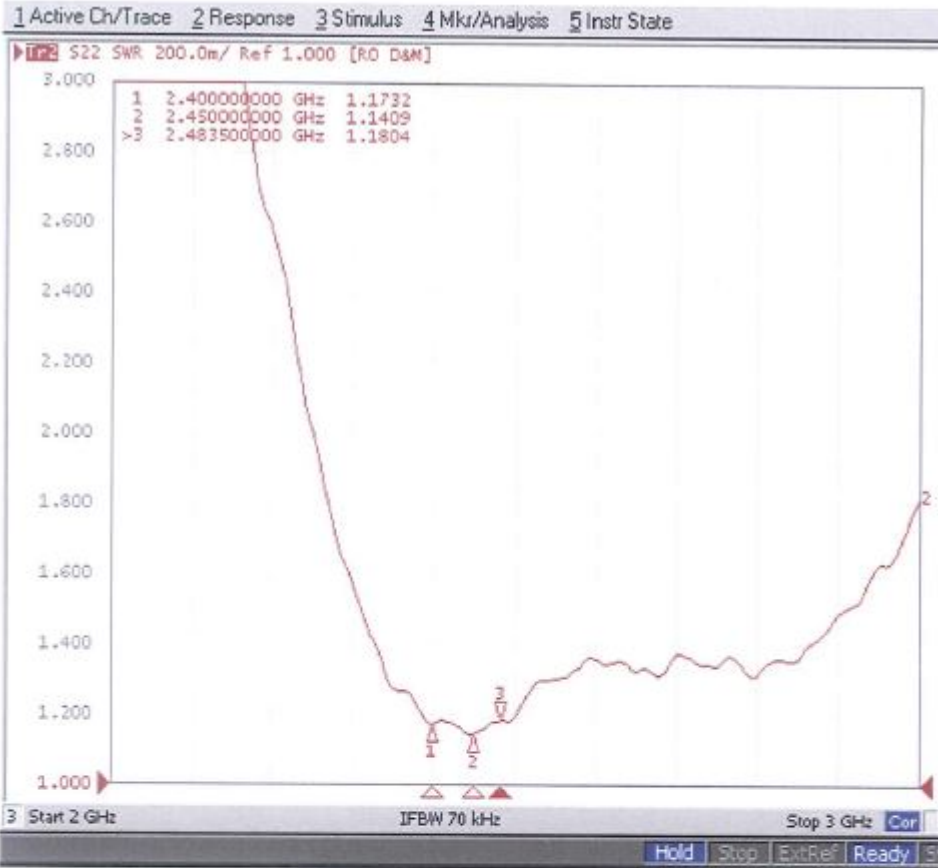
OYH02φ22-NF (Ver. 2)
