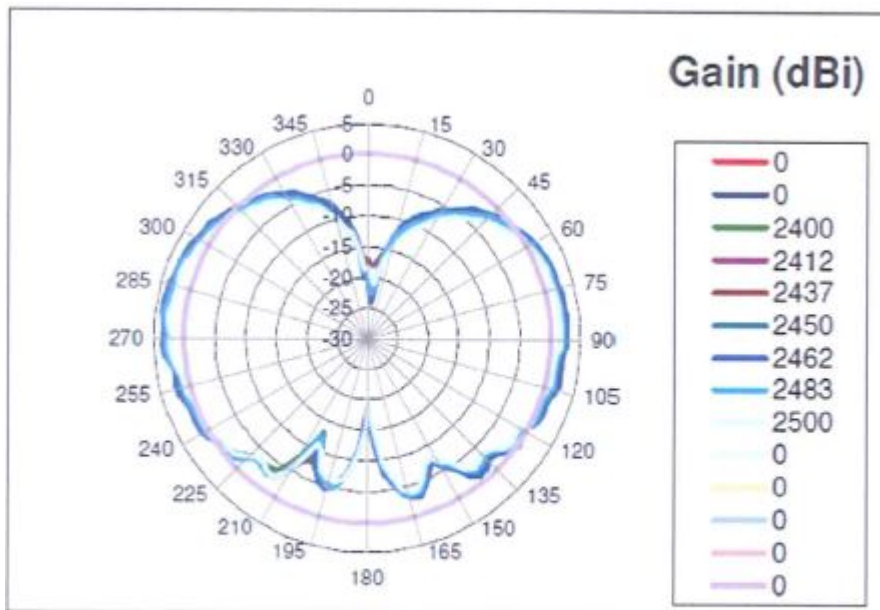
OYH02φ22-NF (Ver. 2)
