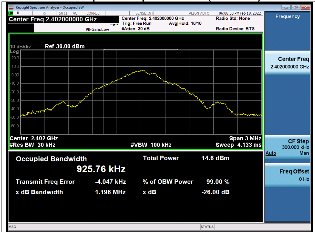
Test_Graph_GFSK_ANT1_2402_OBW
