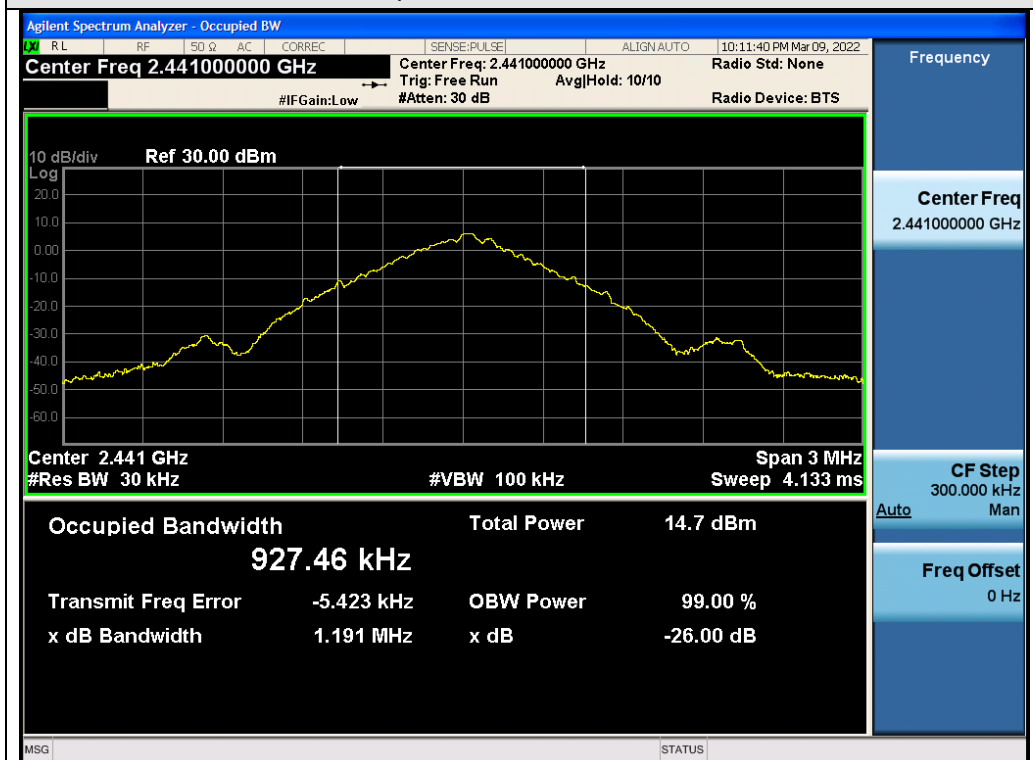
Test_Graph_GFSK_ANT1_2441_OBW
