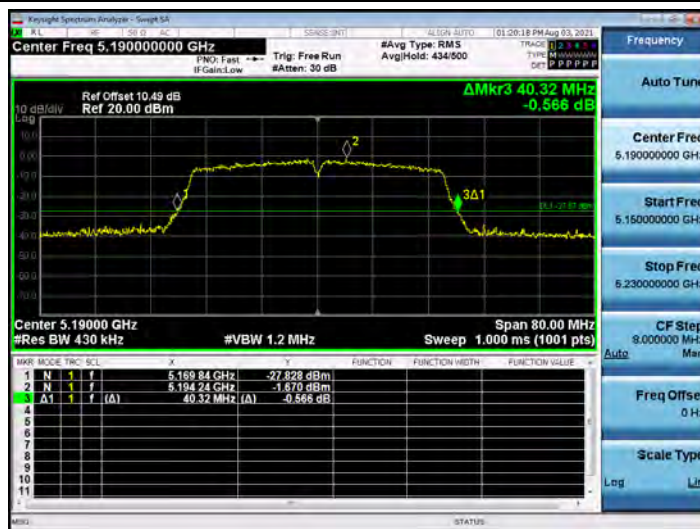
802.11ac VHT40_5190
