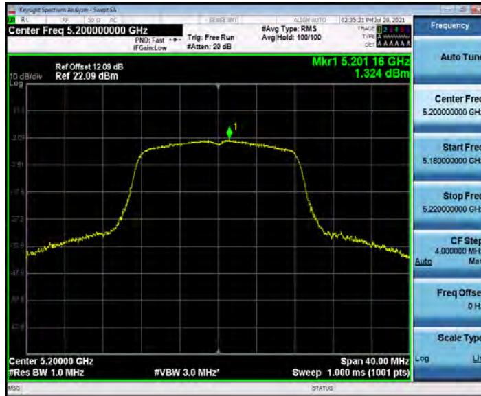
802.11a_5200
