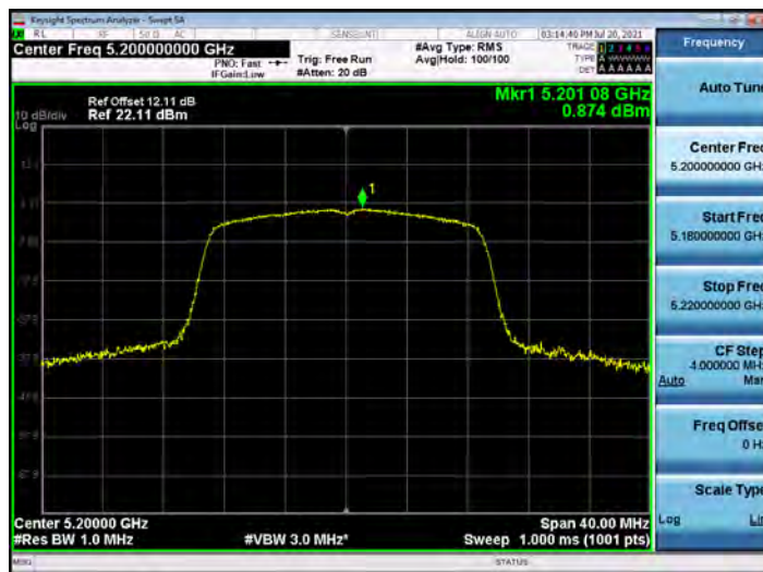
802.11ac VHT20_5200
