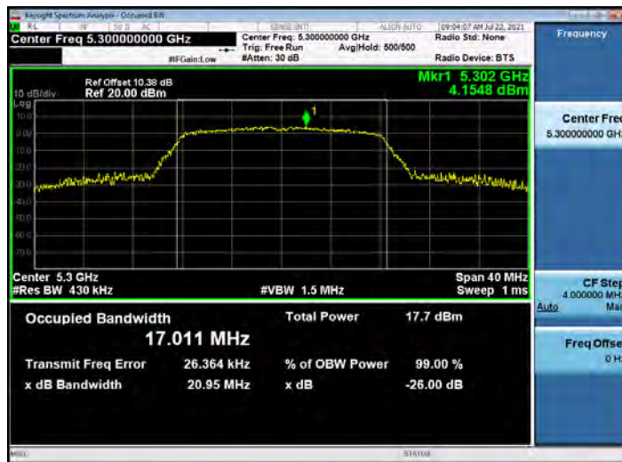
802.11a_5300
