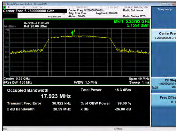
802.11ac VHT20_5260
