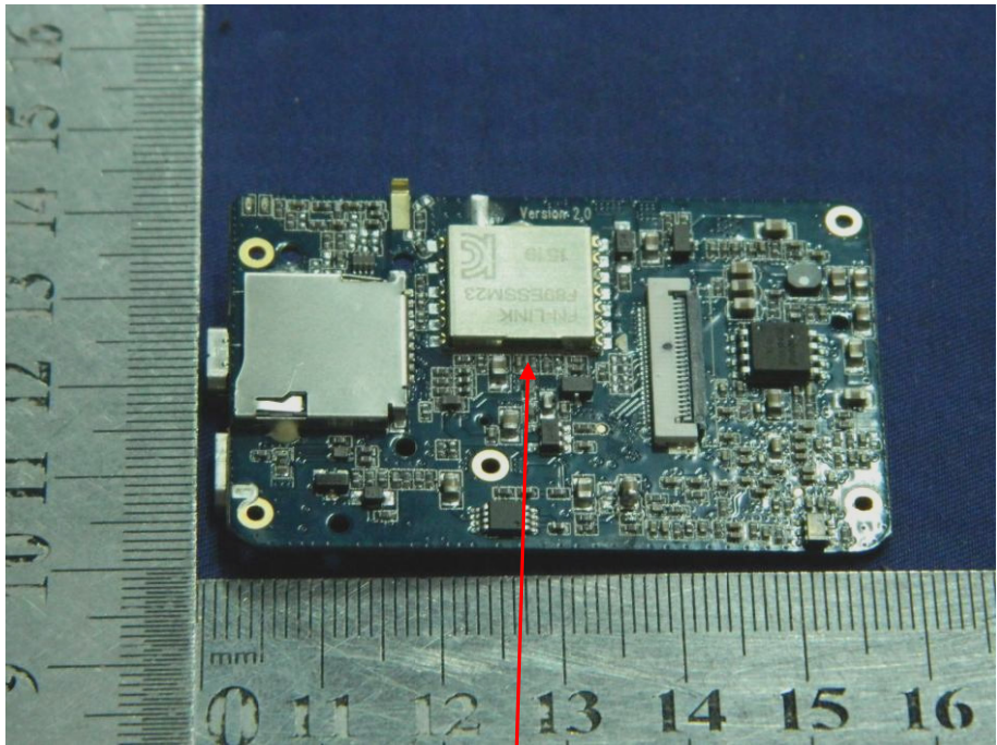
WIFI Module
