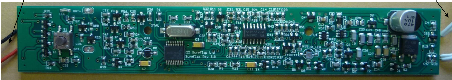
PCB top
