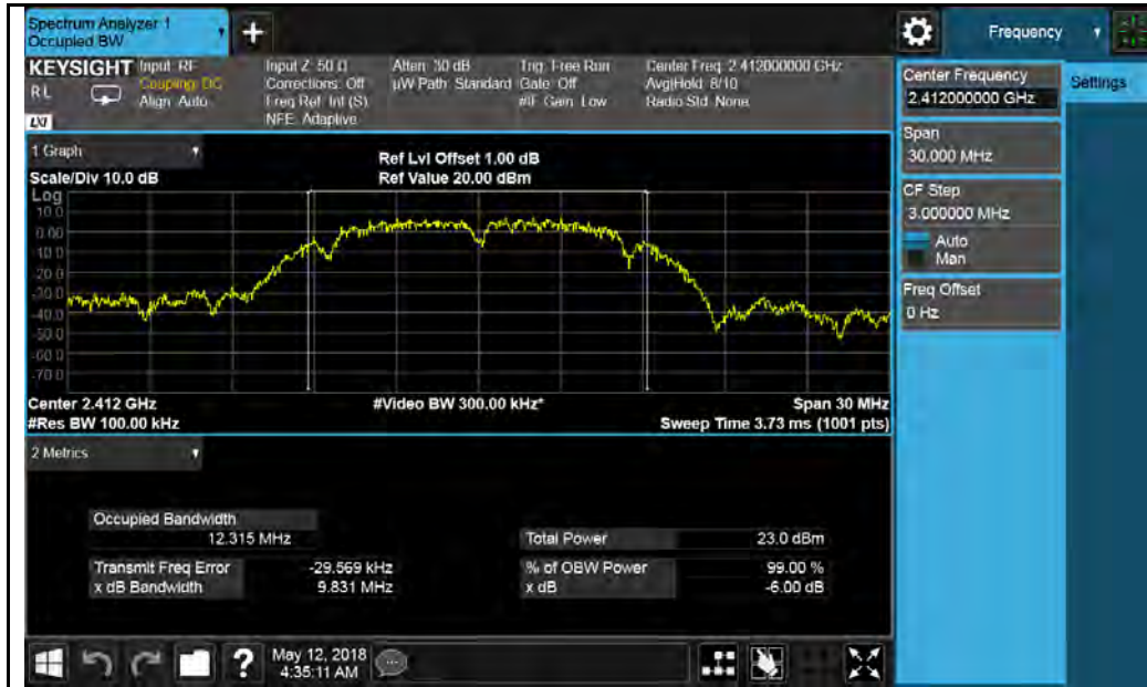
802.11b-2412MHz
