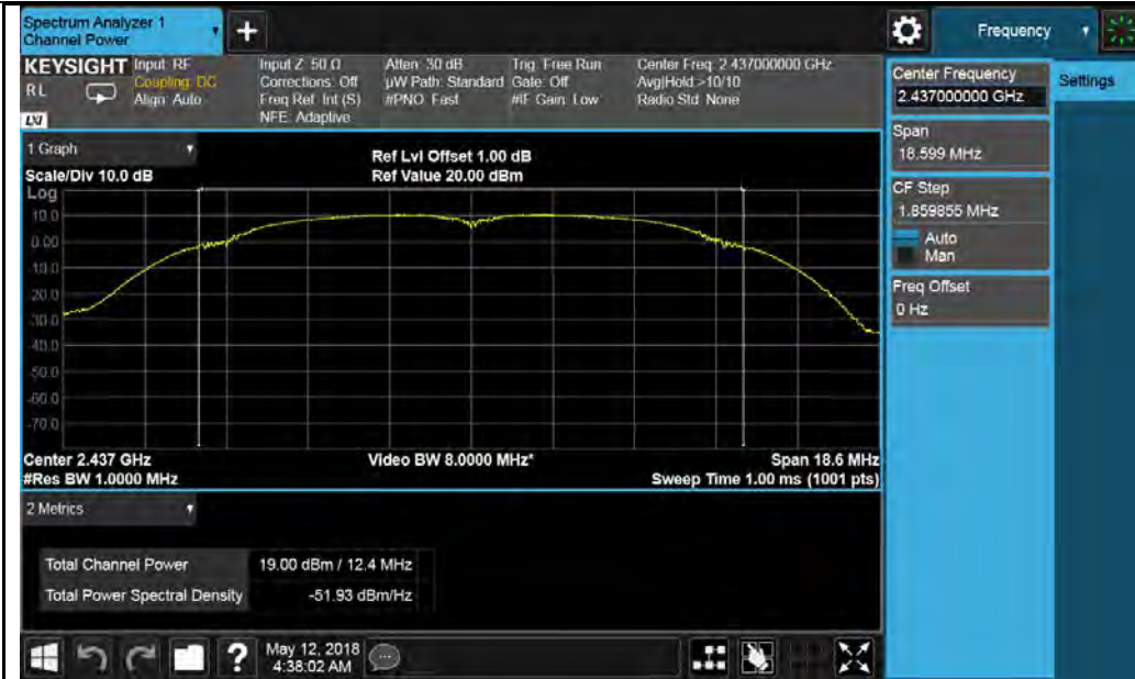
802.11b-2437MHz Chain 0
