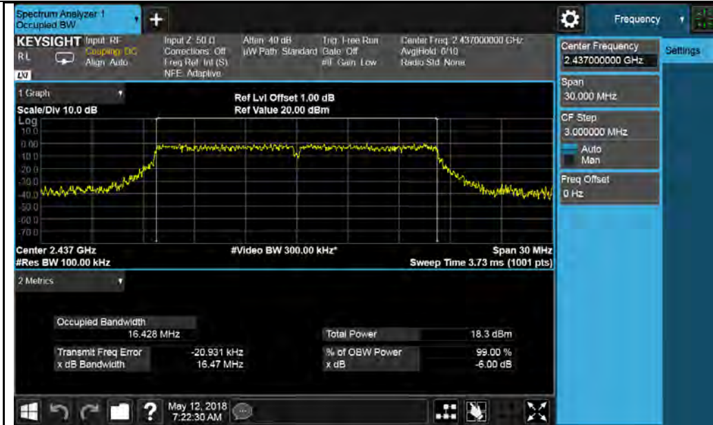
802.11g-2437MHz
