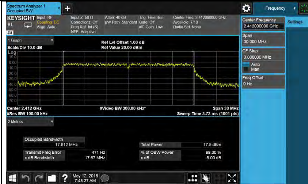
802.11n-HT20-2412MHz
