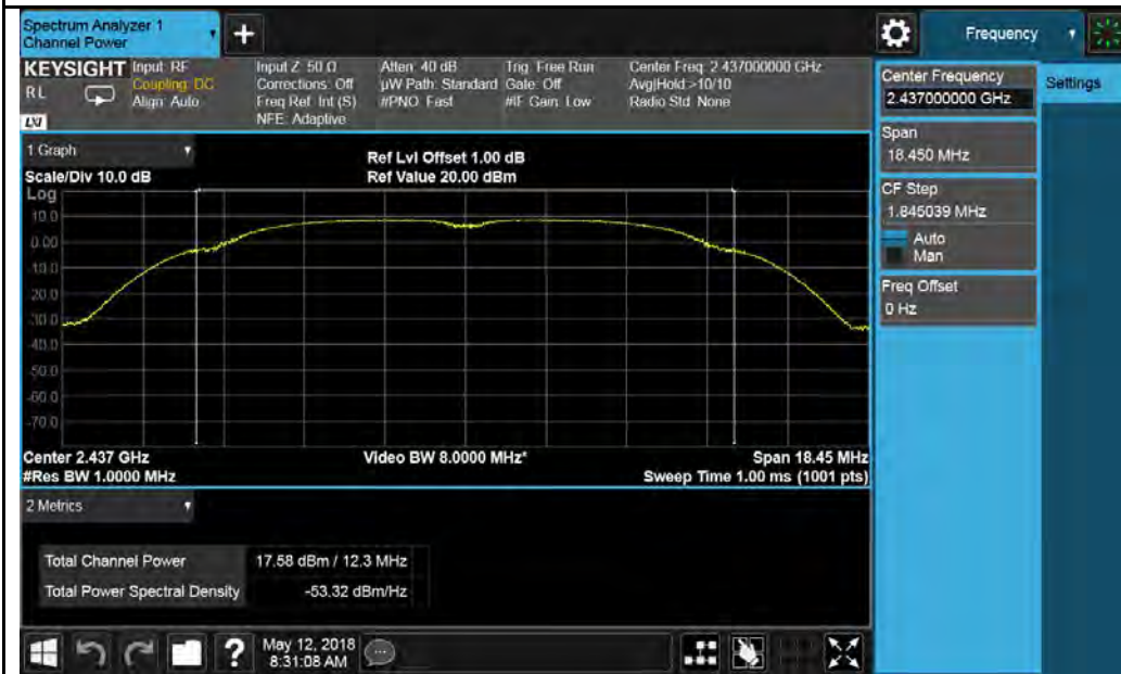
802.11b-2437MHz Chain 1
