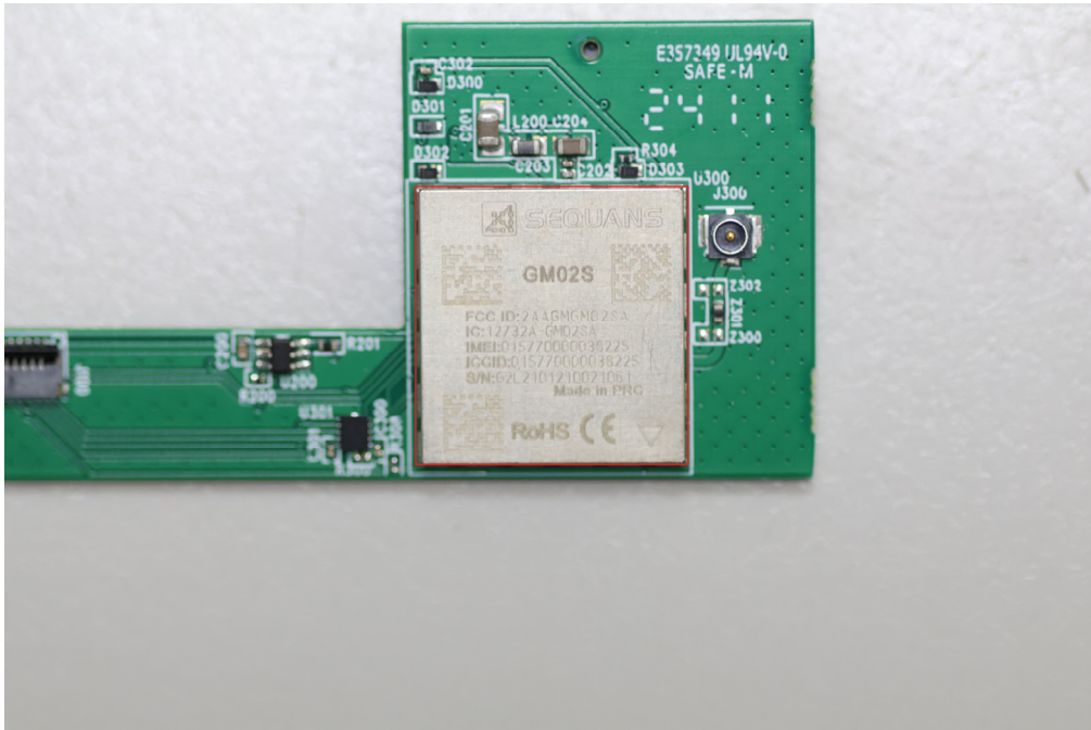
WWAN RFIC
