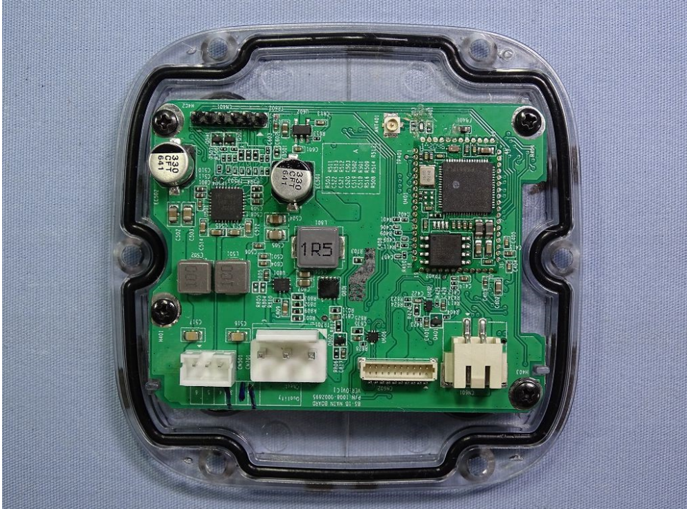
(4) EUT Photo
