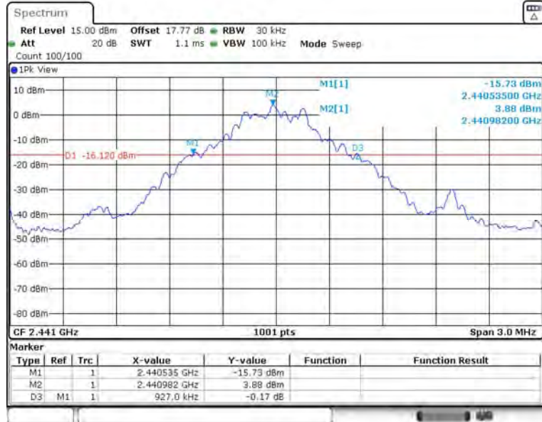
DH5_Ant1_2441
