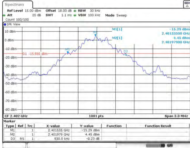
DH5_Ant1_2402
