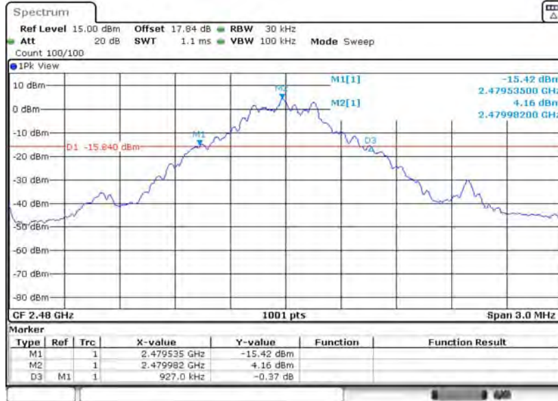
DH5_Ant1_2480
