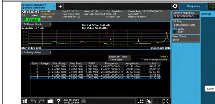
Band7-20MHz-QPSK-20850-1RB#99-PASS
