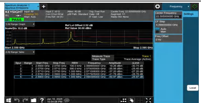
Band7-20MHz-QPSK-21350-1RB#99-PASS
