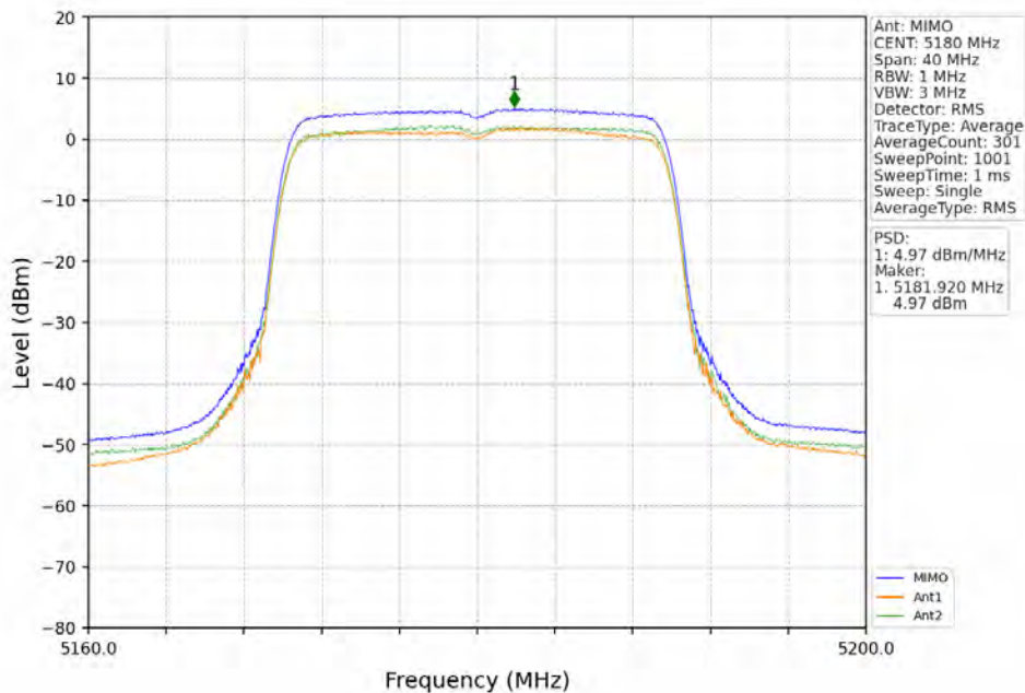
802.11ax(HE20)_LCH_5180MHz_RU242_Left_MIMO_NTNV
