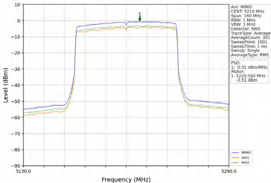
802.11ax(HE80)_MCH_5210MHz_RU996_Left_MIMO_NTNV
