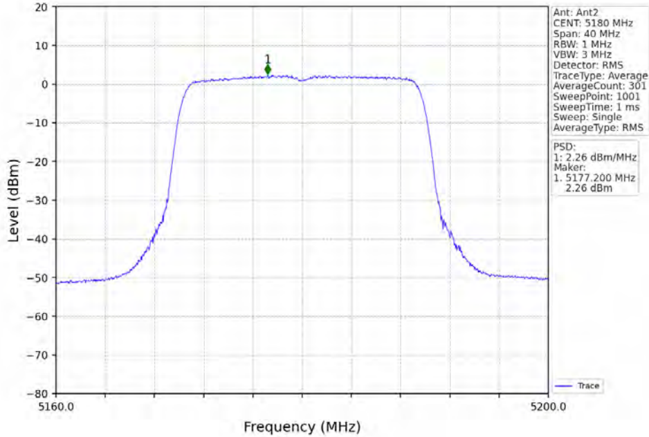
802.11ax(HE20)_LCH_5180MHz_RU242_Left_MIMO_NTNV
