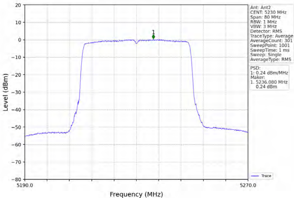
802.11ax(HE40)_HCH_5230MHz_RU484_Left_Ant2_NTNV
