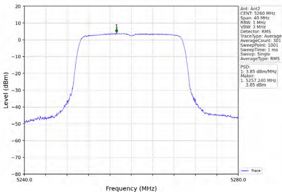
802.11ax(HE20)_LCH_5260MHz_RU242_Left_Ant2_NTNV
