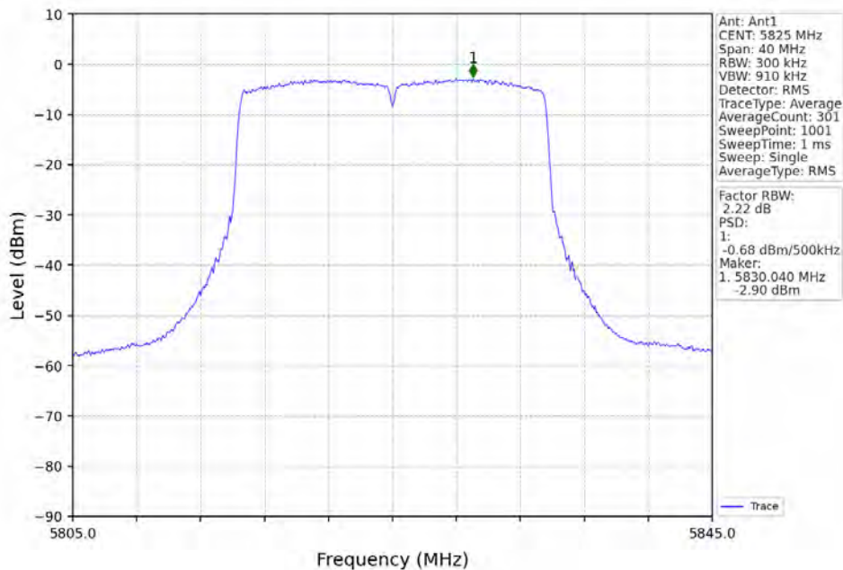
802.11ax(HE20)_HCH_5825MHz_RU242_Left_Ant1_NTNV
