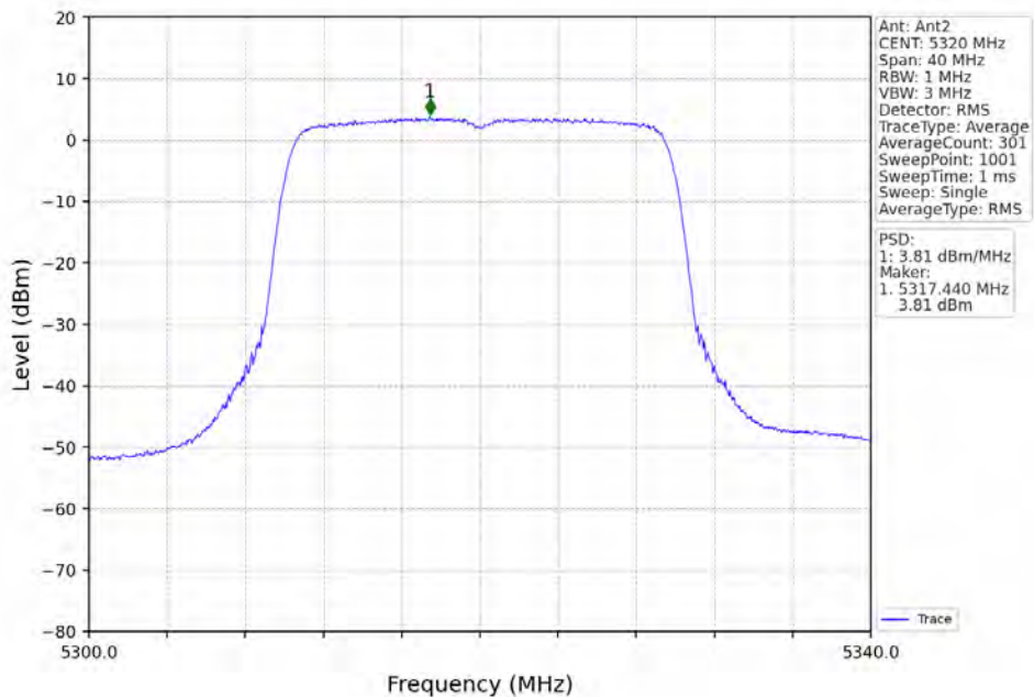
802.11ax(HE20)_HCH_5320MHz_RU242_Left_Ant2_NTNV
