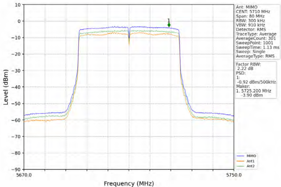
802.11ax(HE40)_HCH_5710MHz_RU484_Left_MIMO_NTNV
