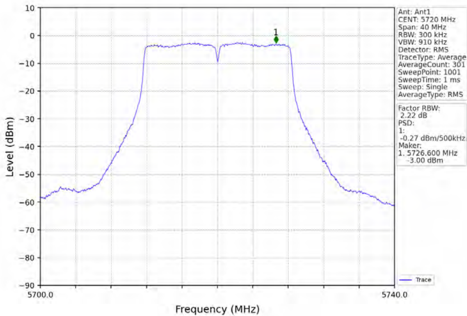
802.11a_HCH_5720MHz_Ant1_NTNV
