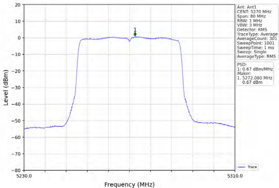
802.11ax(HE40)_LCH_5270MHz_RU484_Left_Ant1_NTNV
