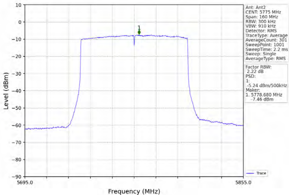
802.11ax(HE80)_MCH_5775MHz_RU996_Left_Ant2_NTNV
