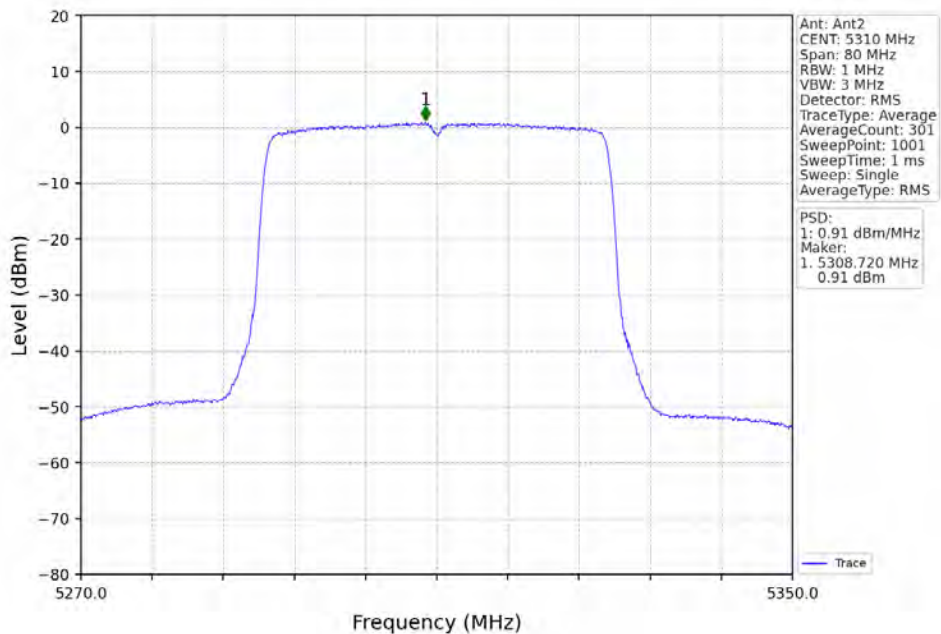
802.11ax(HE40)_HCH_5310MHz_RU484_Left_Ant2_NTNV
