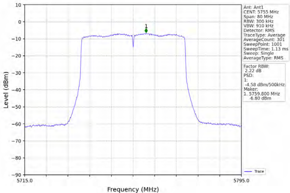
802.11ax(HE40)_LCH_5755MHz_RU484_Left_Ant1_NTNV
