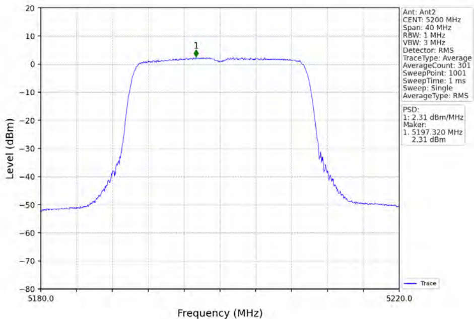
802.11ax(HE20)_MCH_5200MHz_RU242_Left_Ant2_NTNV
