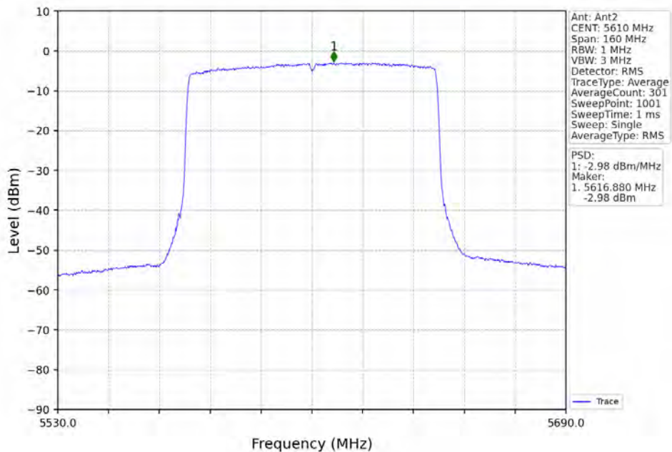
802.11ax(HE80)_HCH_5610MHz_RU996_Left_Ant2_NTNV
