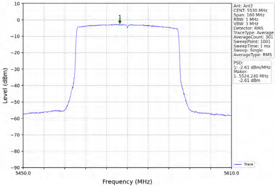
802.11ax(HE80)_LCH_5530MHz_RU996_Left_MIMO_NTNV
