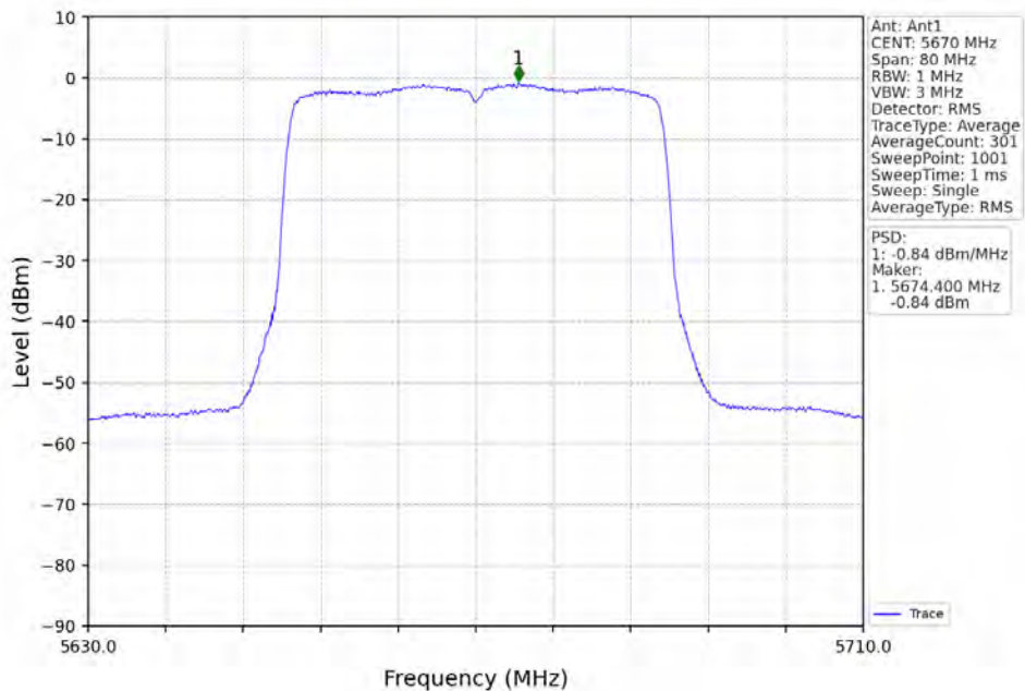
802.11ax(HE40)_HCH_5670MHz_RU484_Left_Ant1_NTNV
