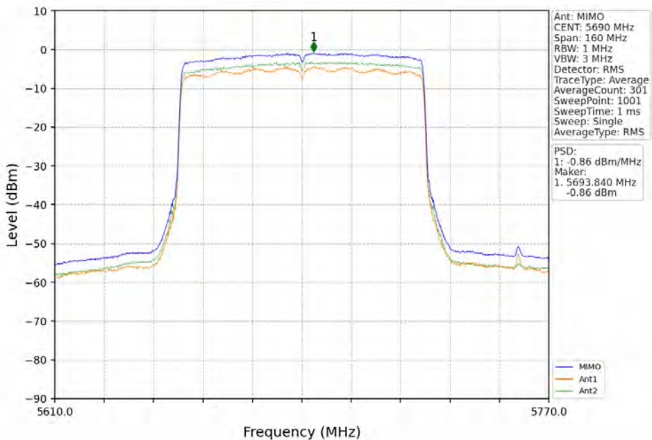
802.11ax(HE80)_HCH_5690MHz_RU996_Left_MIMO_NTNV
