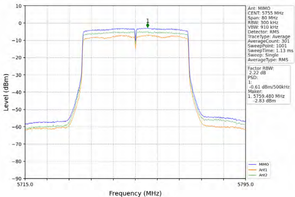
802.11ax(HE40)_LCH_5755MHz_RU484_Left_MIMO_NTNV
