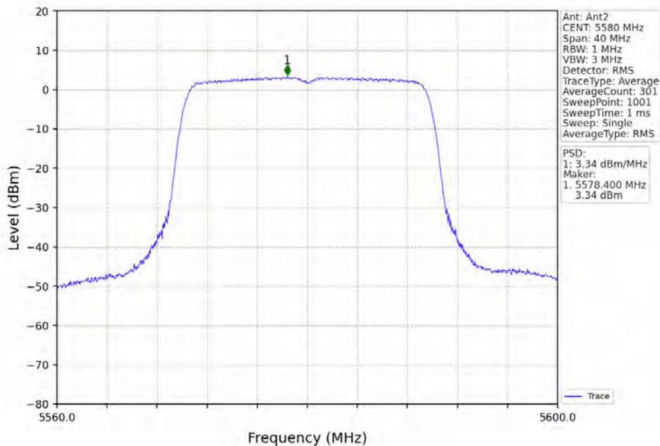
802.11ax(HE20)_MCH_5580MHz_RU242_Left_Ant2_NTNV
