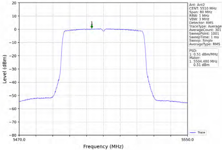
802.11ax(HE40)_LCH_5510MHz_RU484_Left_MIMO_NTNV
