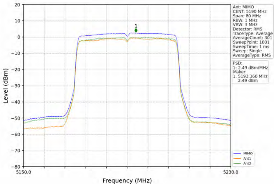
802.11ax(HE40)_LCH_5190MHz_RU484_Left_MIMO_NTNV
