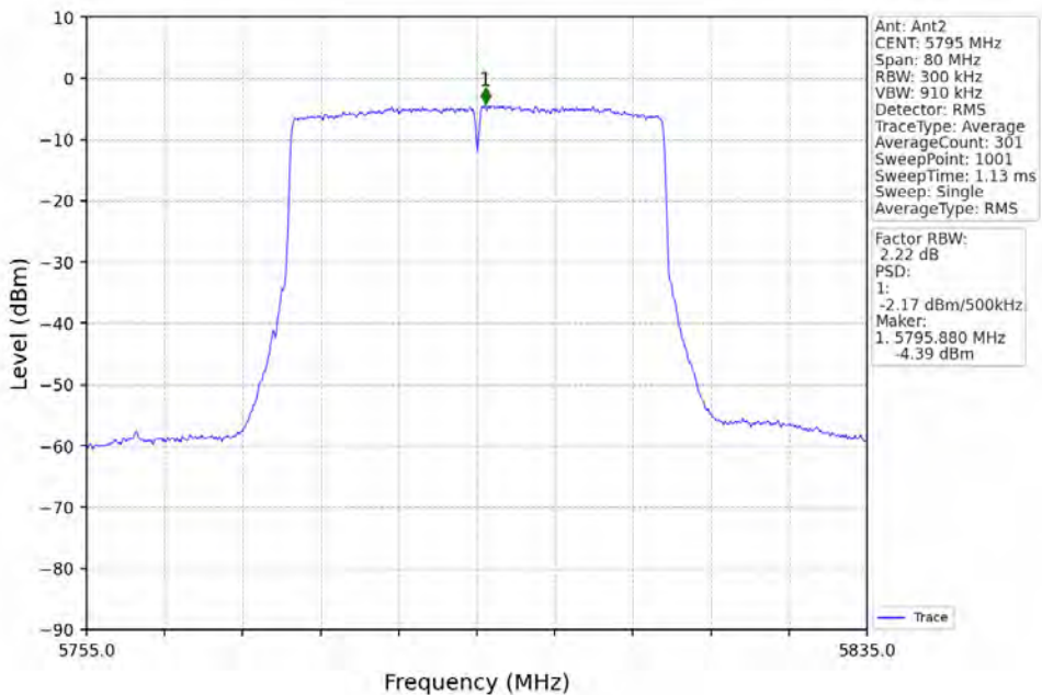
802.11ax(HE40)_HCH_5795MHz_RU484_Left_Ant2_NTNV
