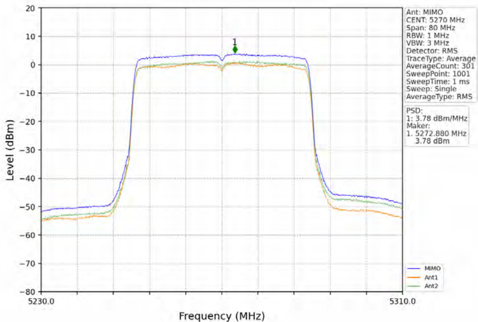
802.11ax(HE40)_LCH_5270MHz_RU484_Left_MIMO_NTNV
