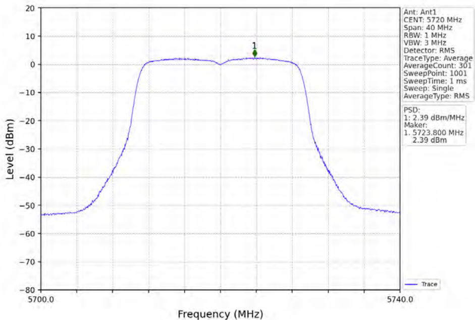
802.11n(HT20)_HCH_5720MHz_Ant1_NTNV
