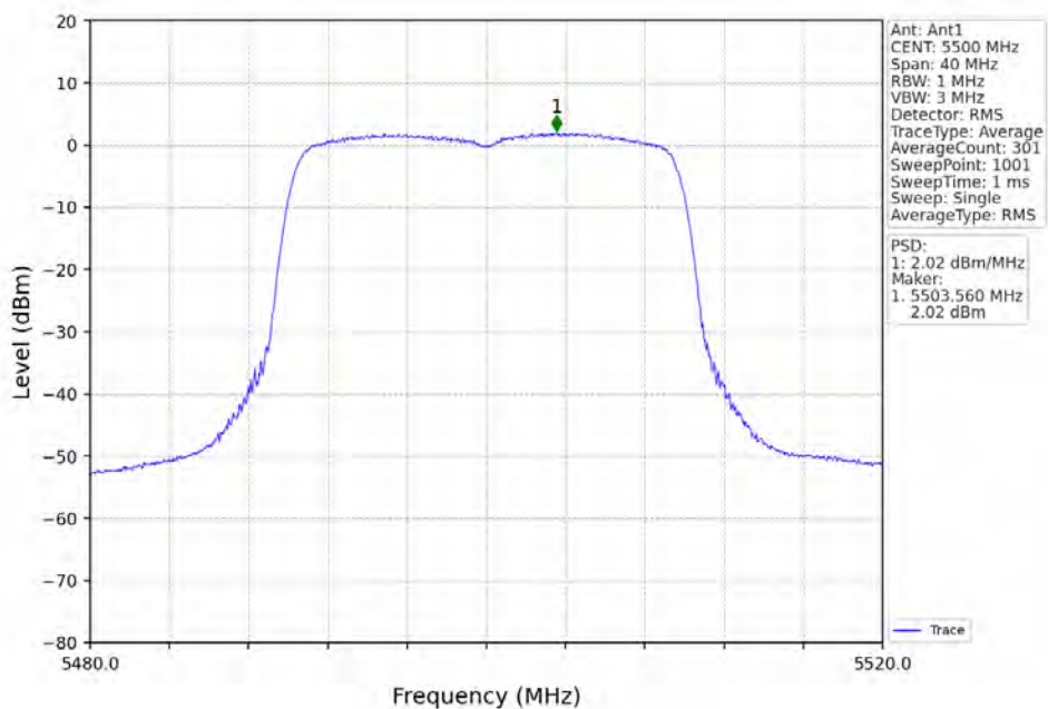
802.11ax(HE20)_LCH_5500MHz_RU242_Left_Ant1_NTNV
