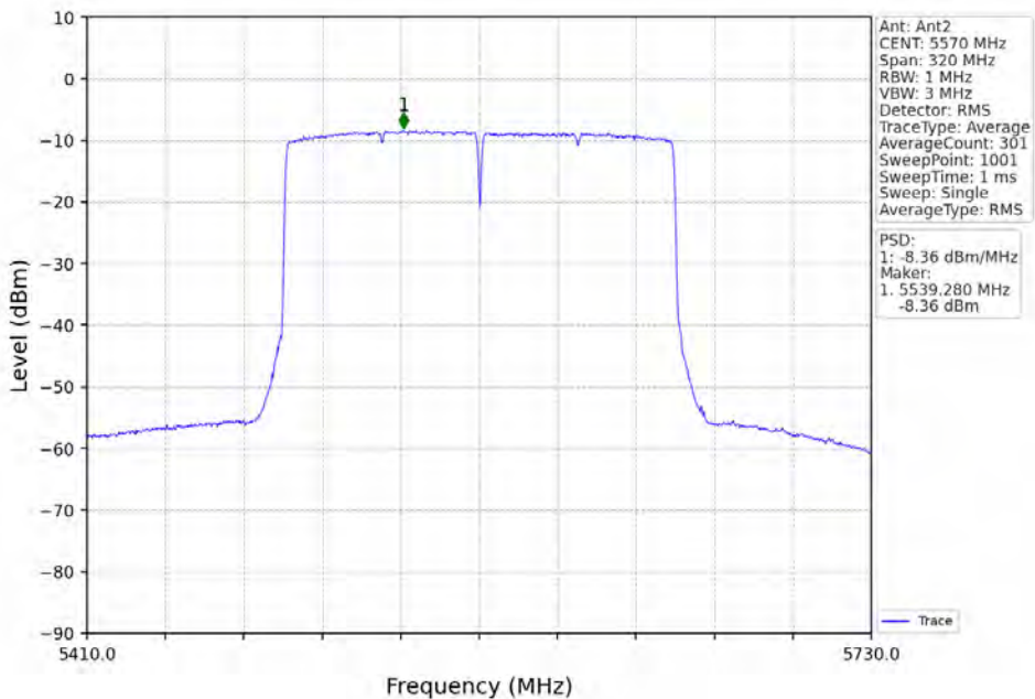
802.11ax(HE160)_MCH_5570MHz_2xRU996_Left_Ant2_NTNV
