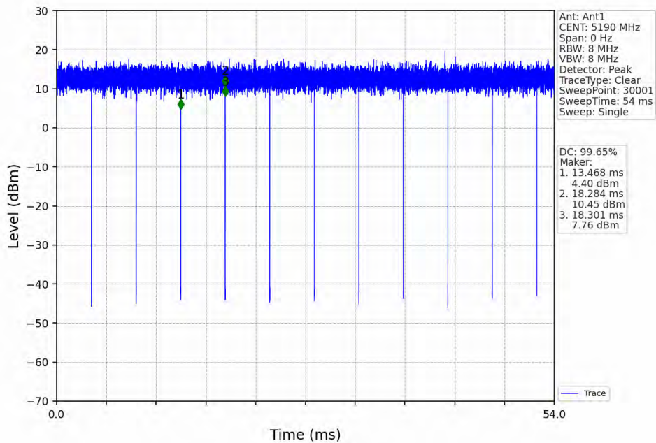
802.11ax(HE40)_LCH_5190MHz_RU484_Left_Ant1_NTNV
