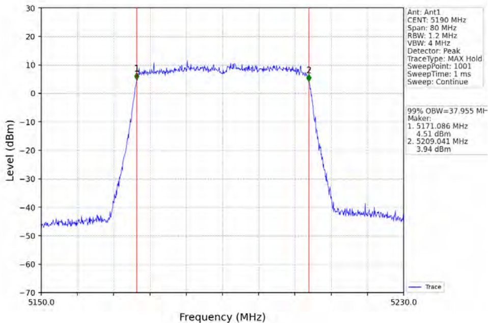
802.11ax(HE40)_LCH_5190MHz_RU484_Left_Ant1_NTNV
