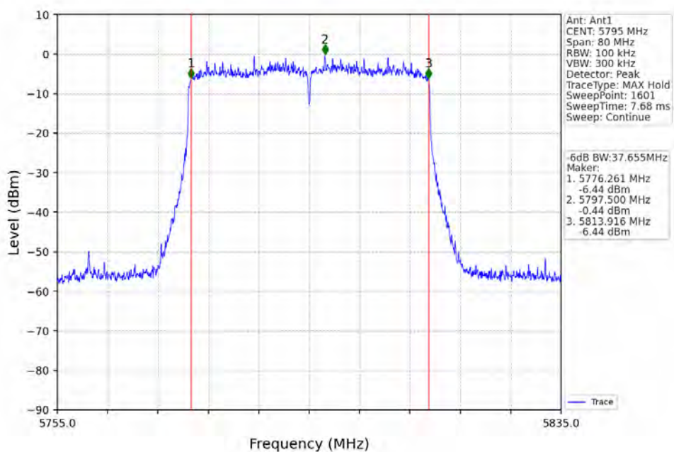
802.11ax(HE40)_HCH_5795MHz_RU484_Left_Ant1_NTNV
