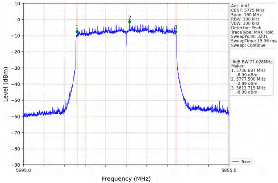
802.11ax(HE80)_MCH_5775MHz_RU996_Left_Ant1_NTNV
