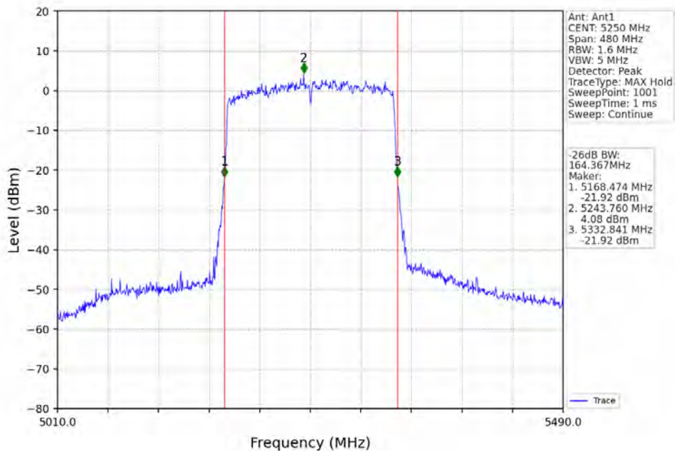
802.11ax(HE160)_MCH_5250MHz_2xRU996_Left_Ant1_NTNV
