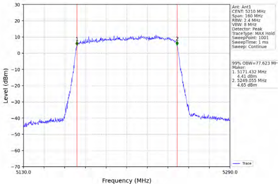
802.11ax(HE80)_MCH_5210MHz_RU996_Left_Ant1_NTNV
