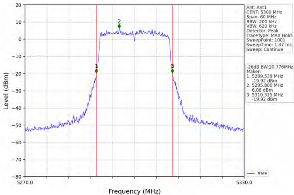
802.11ax(HE20)_MCH_5300MHz_RU242_Left_Ant1_NTNV
