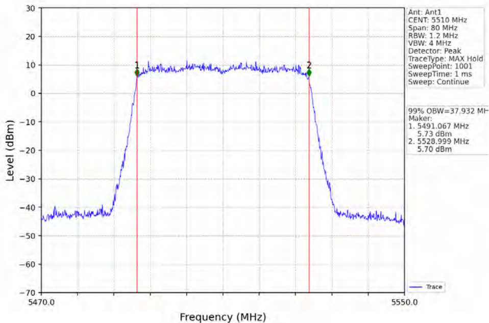
802.11ax(HE40)_LCH_5510MHz_RU484_Left_Ant1_NTNV
