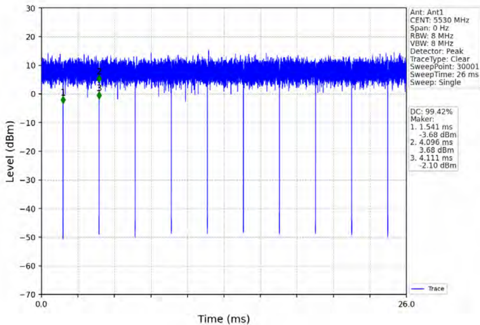
802.11ax(HE80)_LCH_5530MHz_RU996_Left_Ant1_NTNV
