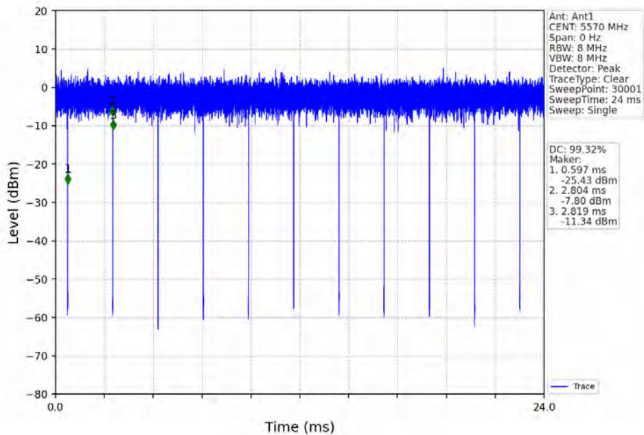
802.11ax(HE160)_MCH_5570MHz_2xRU996_Left_Ant1_NTNV
