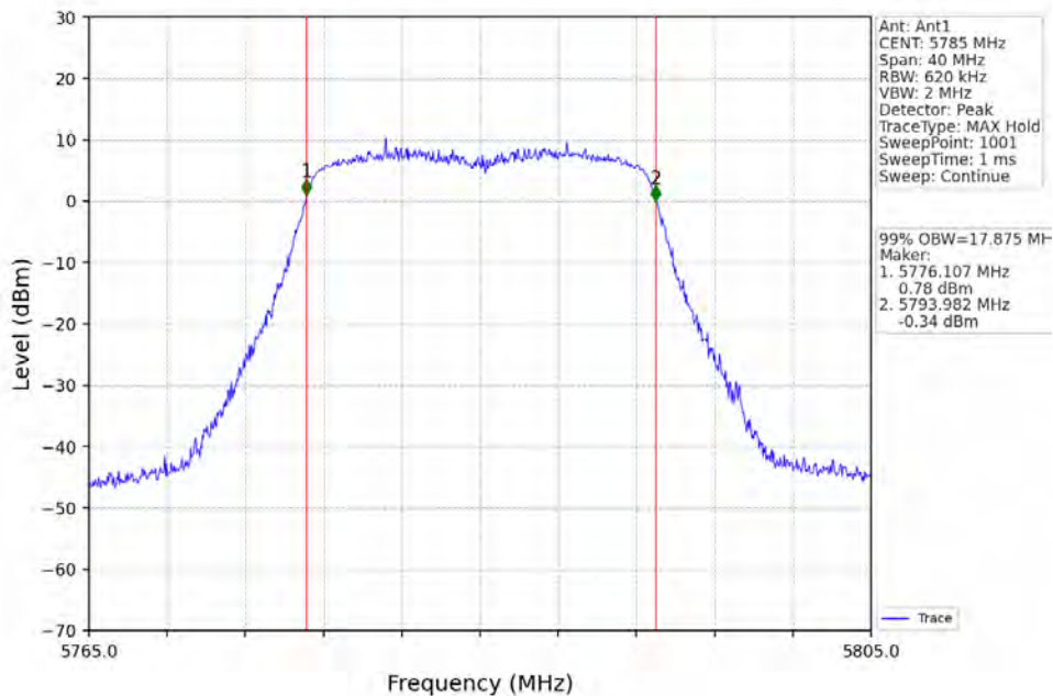
802.11n(HT20)_MCH_5785MHz_Ant1_NTNV
