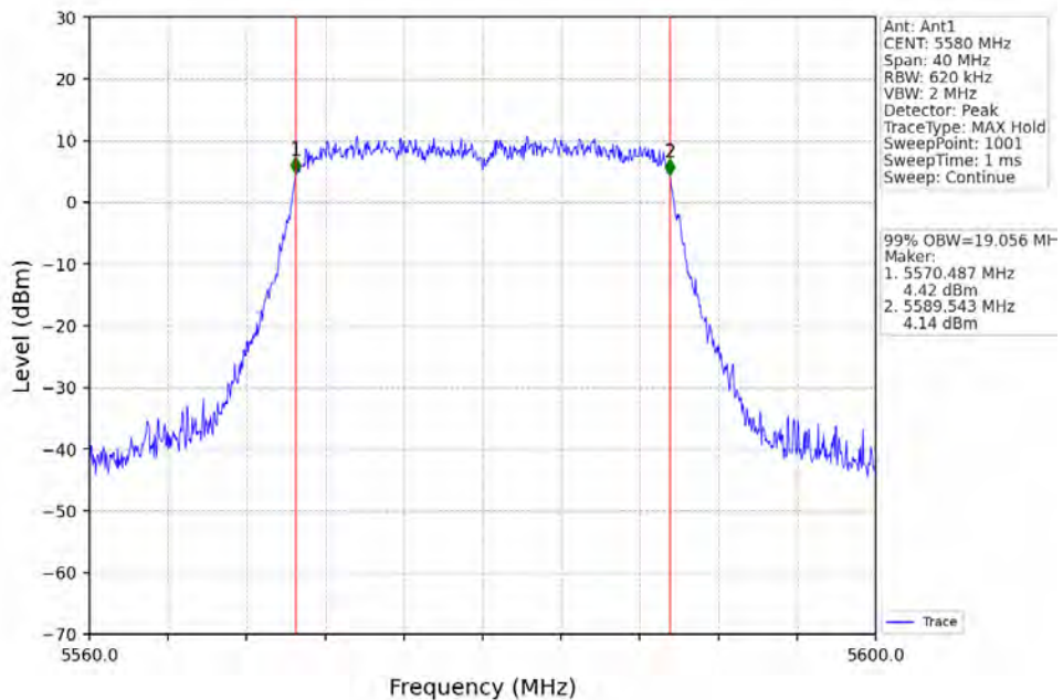
802.11ax(HE20)_MCH_5580MHz_RU242_Left_Ant1_NTNV
