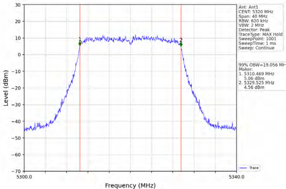
802.11ax(HE20)_HCH_5320MHz_RU242_Left_Ant1_NTNV
