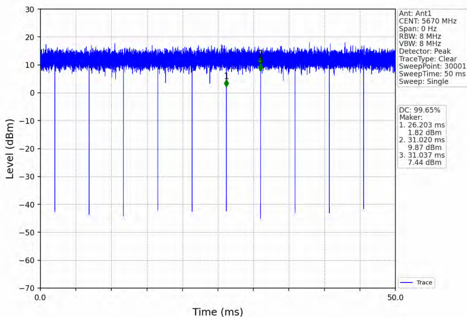
802.11ax(HE40)_HCH_5670MHz_RU484_Left_Ant1_NTNV
