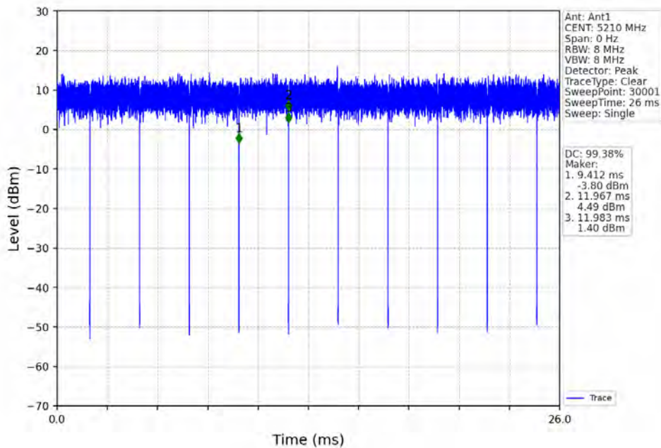
802.11ax(HE80)_MCH_5210MHz_RU996_Left_Ant1_NTNV
