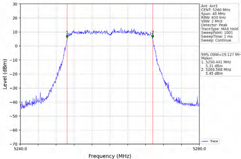
802.11ax(HE20)_LCH_5260MHz_RU242_Left_Ant1_NTNV
