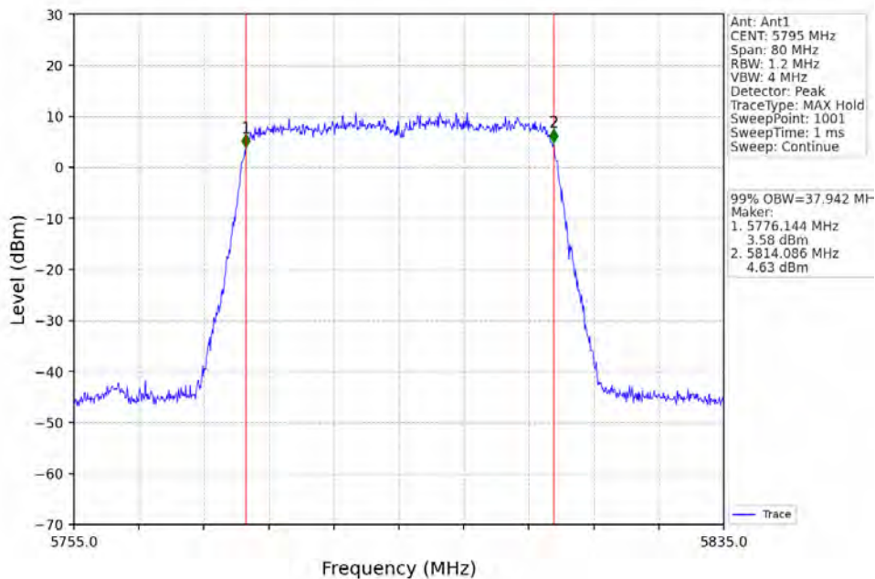
802.11ax(HE40)_HCH_5795MHz_RU484_Left_Ant1_NTNV
