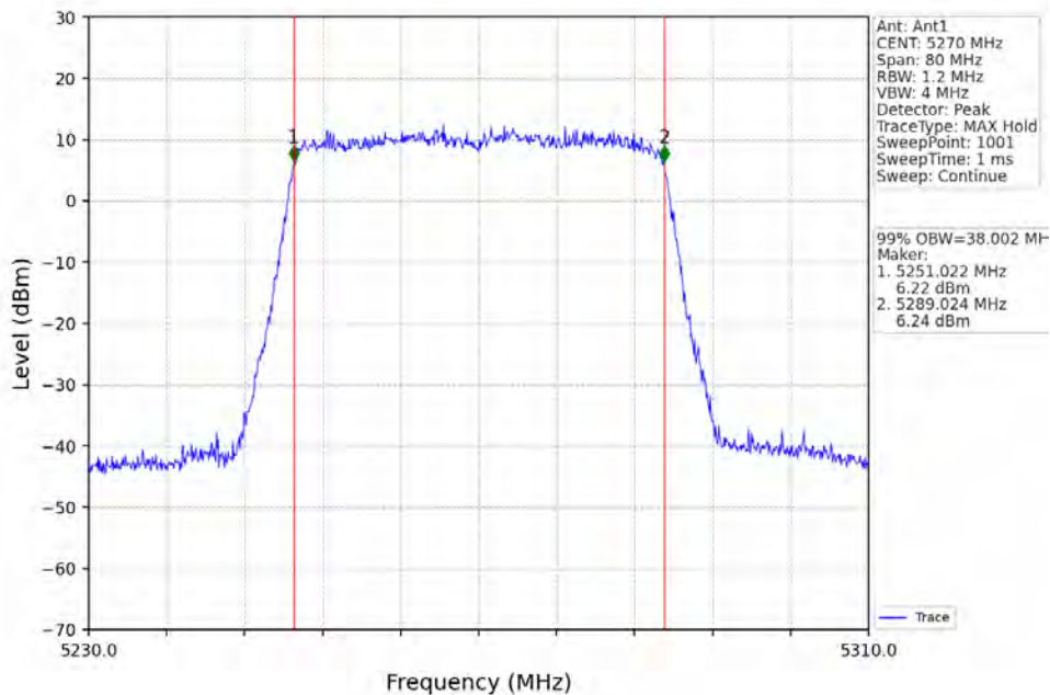
802.11ax(HE40)_LCH_5270MHz_RU484_Left_Ant1_NTNV
