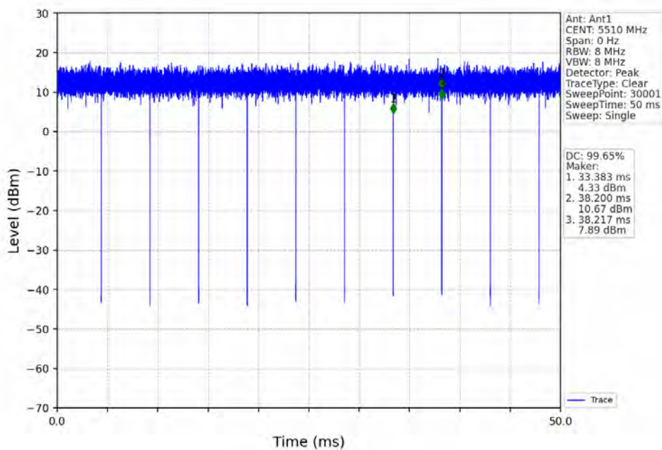
802.11ax(HE40)_LCH_5510MHz_RU484_Left_Ant1_NTNV
