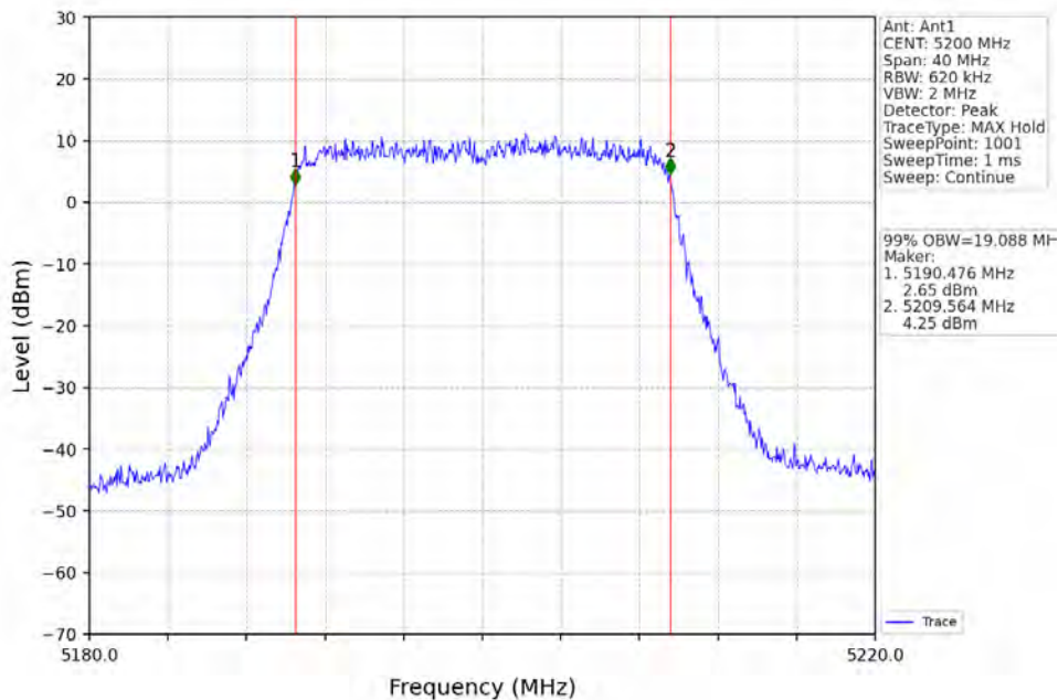
802.11ax(HE20)_MCH_5200MHz_RU242_Left_Ant1_NTNV
