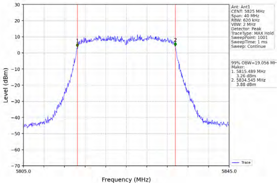
802.11ax(HE20)_HCH_5825MHz_RU242_Left_Ant1_NTNV
