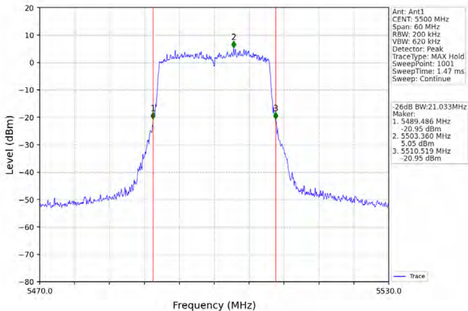
802.11ax(HE20)_LCH_5500MHz_RU242_Left_Ant1_NTNV
