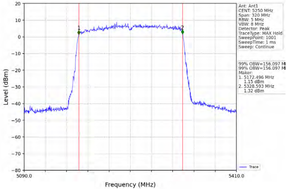
802.11ax(HE160)_MCH_5250MHz_2xRU996_Left_Ant1_NTNV
