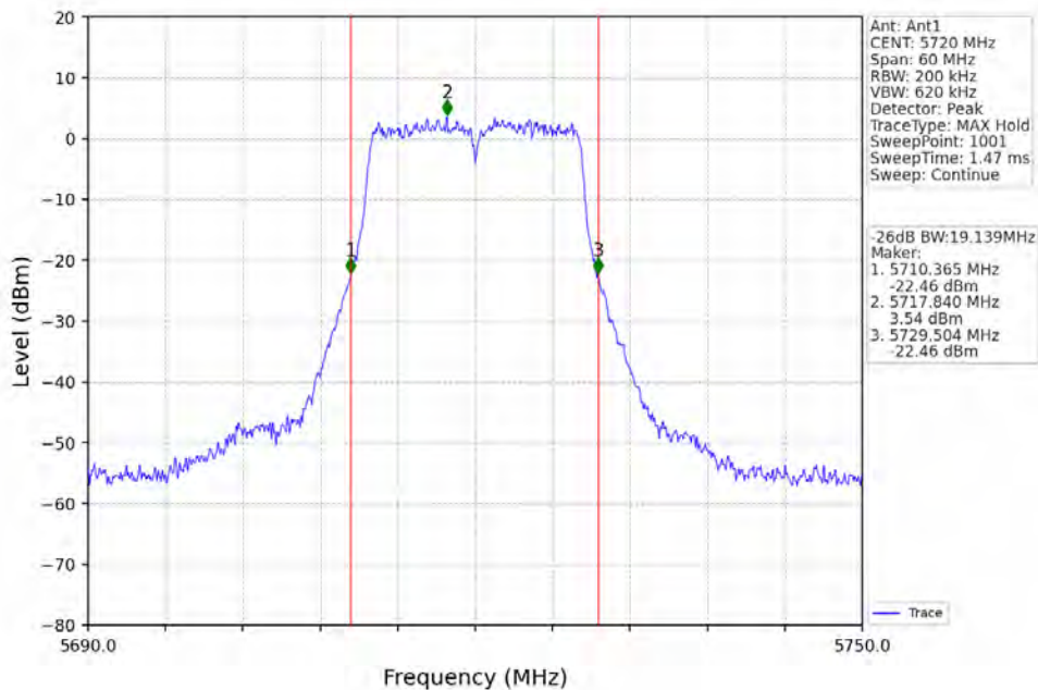
802.11a_HCH_5720MHz_Ant1_NTNV
