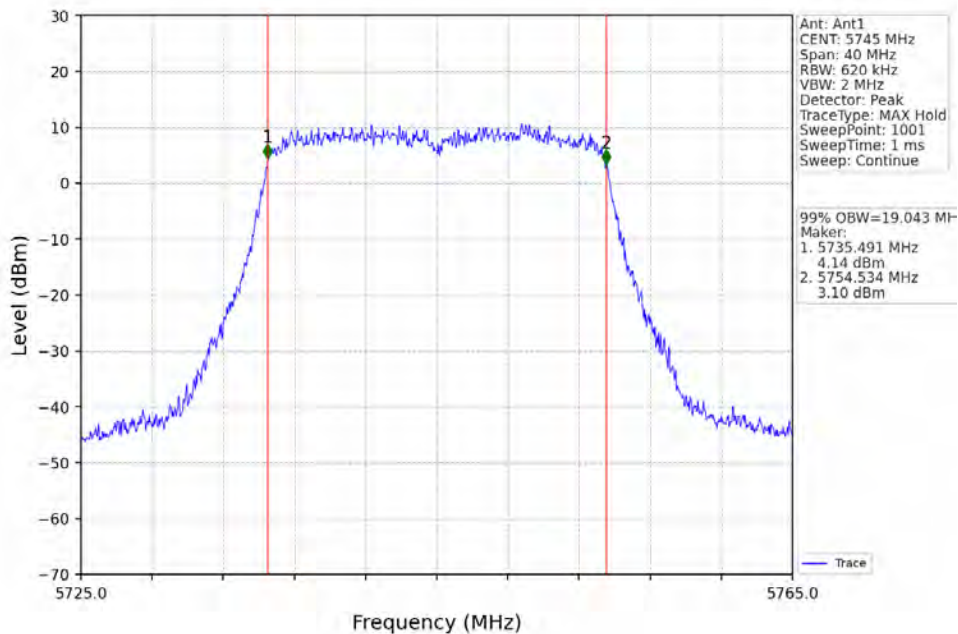
802.11ax(HE20)_LCH_5745MHz_RU242_Left_Ant1_NTNV
