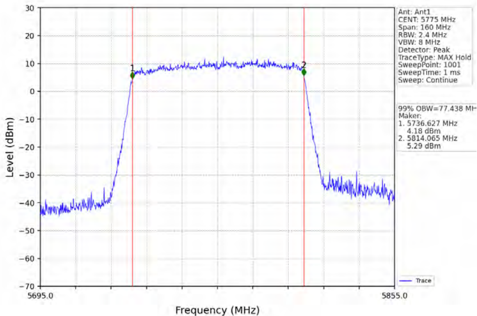
802.11ax(HE80)_MCH_5775MHz_RU996_Left_Ant1_NTNV
