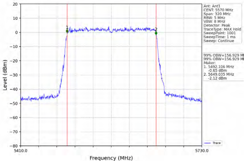
802.11ax(HE160)_MCH_5570MHz_2xRU996_Left_Ant1_NTNV
