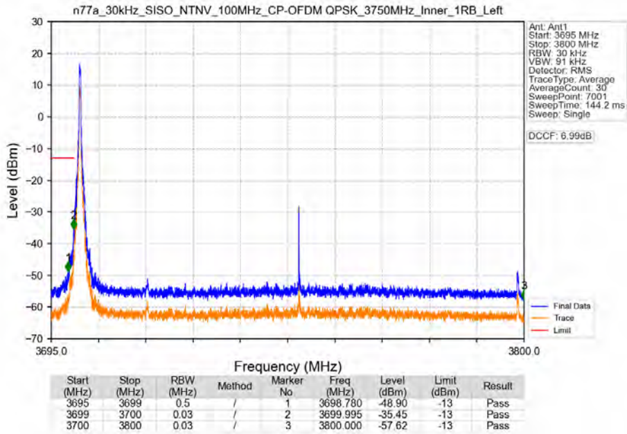
n77a_30kHz_SISO_NTNV_100MHz_CP-OFDM QPSK_3750MHz_Inner_1RB_Left
