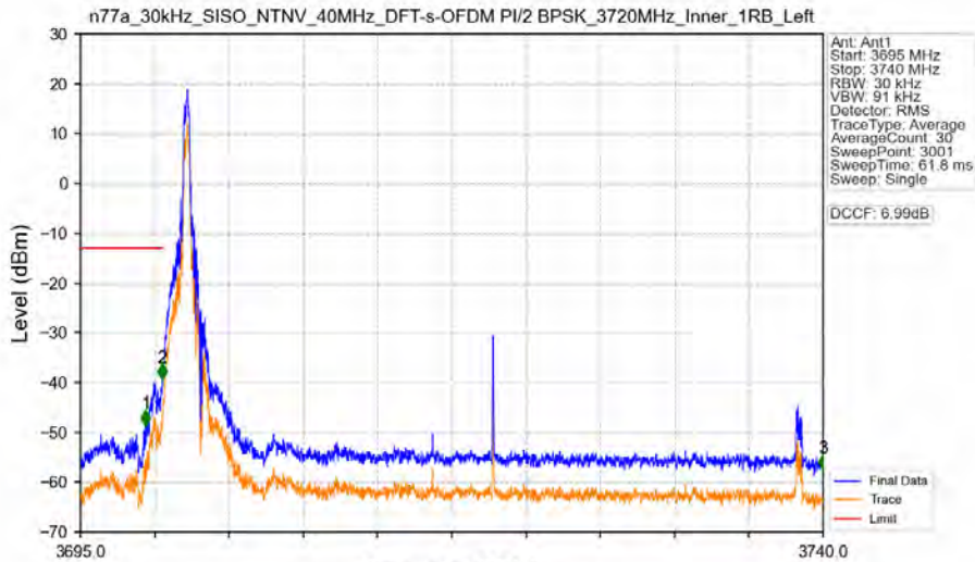
n77a_30kHz_SISO_NTNV_40MHz_DFT-s-OFDM PI/2 BPSK_3720MHz_Inner_1RB_Left
