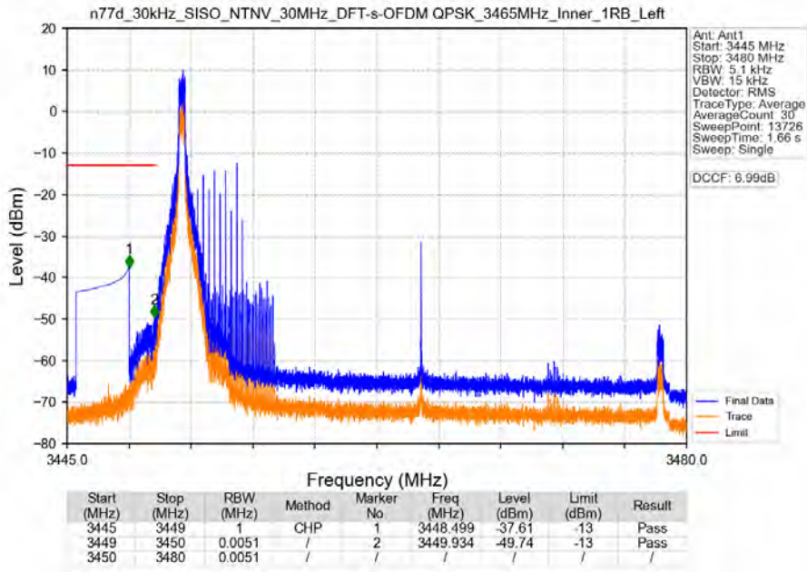
n77d_30kHz_SISO_NTNV_30MHz_DFT-s-OFDM QPSK_3465MHz_Inner_1RB_Left
