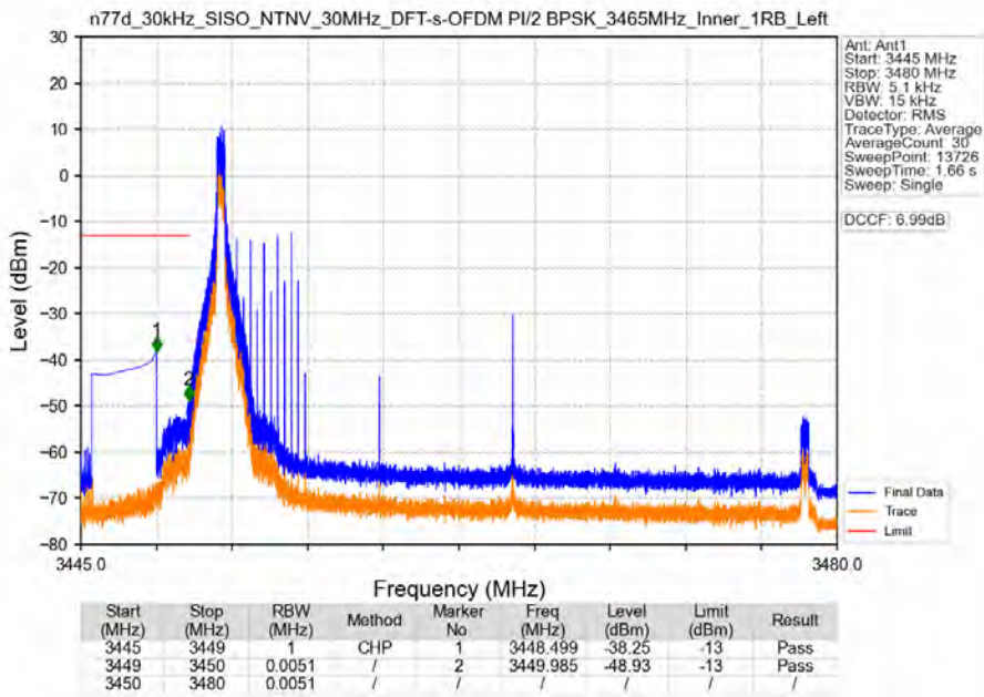
n77d_30kHz_SISO_NTNV_30MHz_DFT-s-OFDM PI/2 BPSK_3465MHz_Inner_1RB_Left
