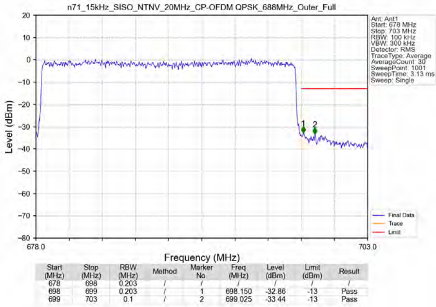
n71_15kHz_SISO_NTNV_20MHz_CP-OFDM QPSK_688MHz_Outer_Full
