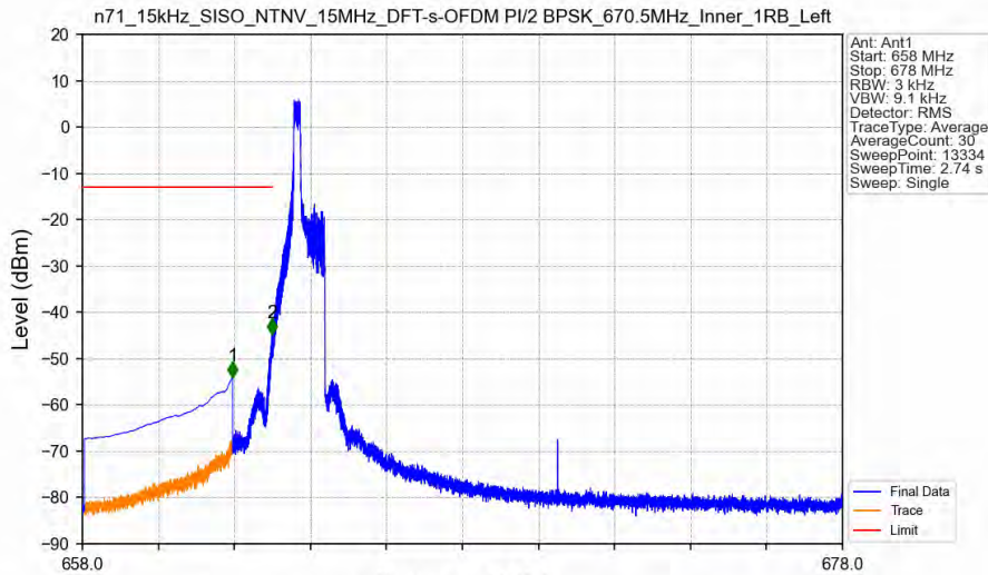
n71_15kHz_SISO_NTNV_15MHz_DFT-s-OFDM PI/2 BPSK_670.5MHz_Inner_1RB_Left
