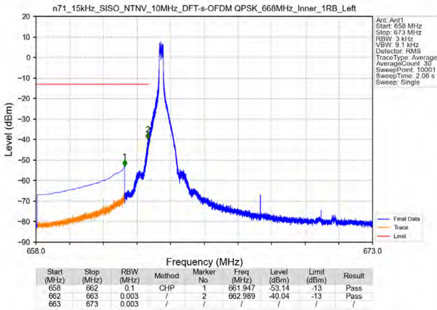
n71_15kHz_SISO_NTNV_10MHz_DFT-s-OFDM QPSK_668MHz_Inner_1RB_Left
