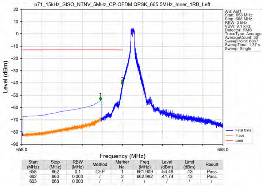
n71_15kHz_SISO_NTNV_5MHz_CP-OFDM QPSK_665.5MHz_Inner_1RB_Left
