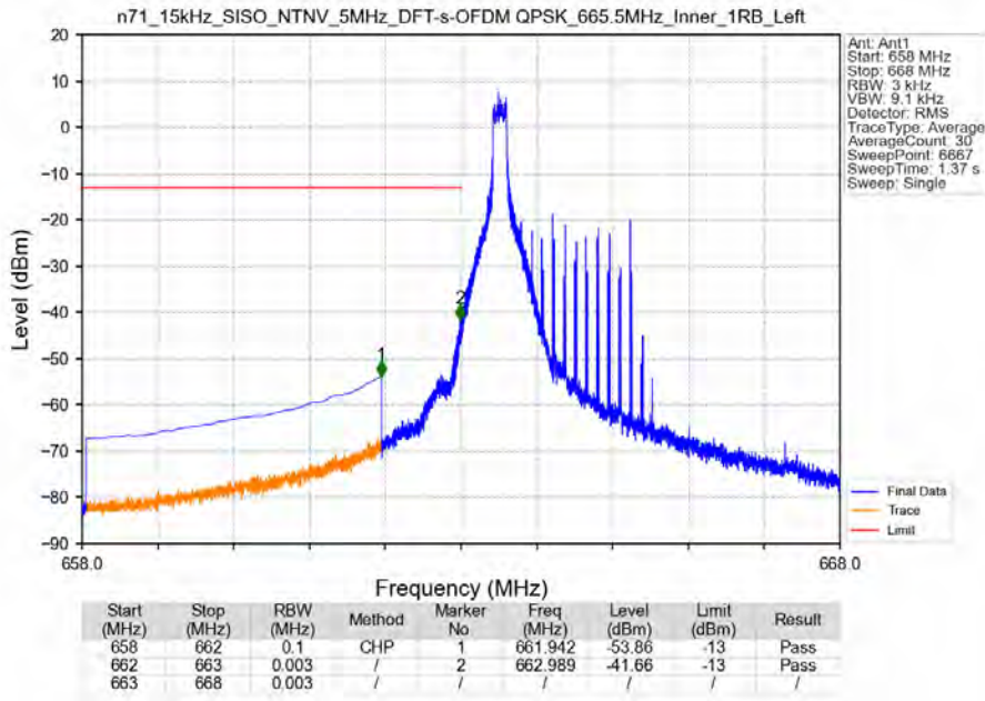
n71_15kHz_SISO_NTNV_5MHz_DFT-s-OFDM_QPSK_665.5MHz_Inner_1RB_Left
