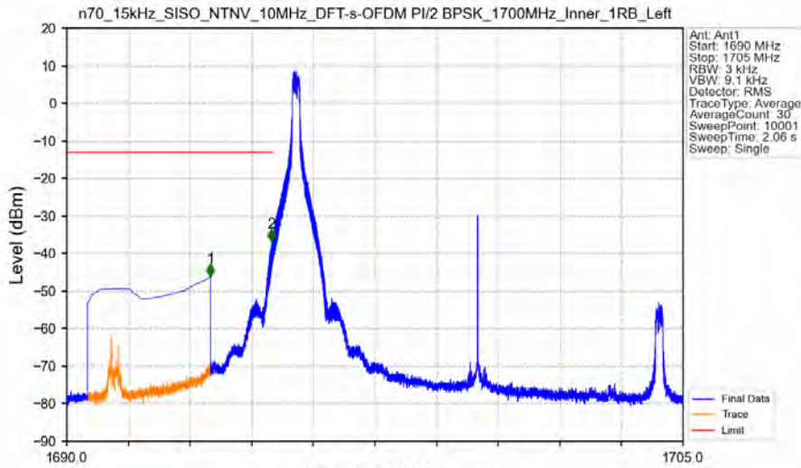
n70_15kHz_SISO_NTNV_10MHz_DFT-s-OFDM PI/2 BPSK_1700MHz_Inner_1RB_Left
