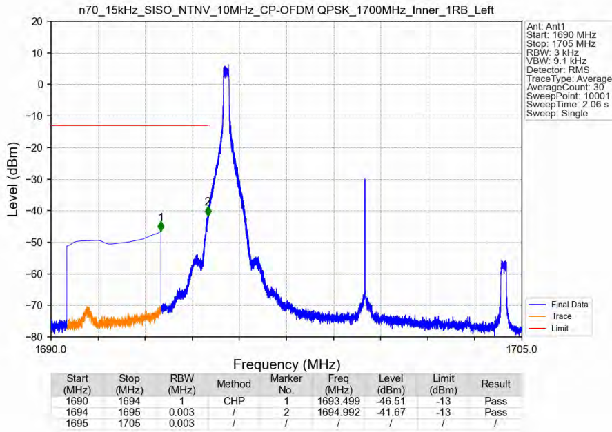
n70_15kHz_SISO_NTNV_10MHz_CP-OFDM QPSK_1700MHz_Inner_1RB_Left
