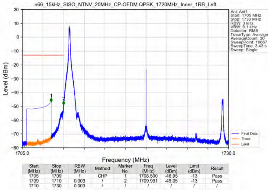
n66_15kHz_SISO_NTNV_20MHz_CP-OFDM QPSK_1720MHz_Inner_1RB_Left
