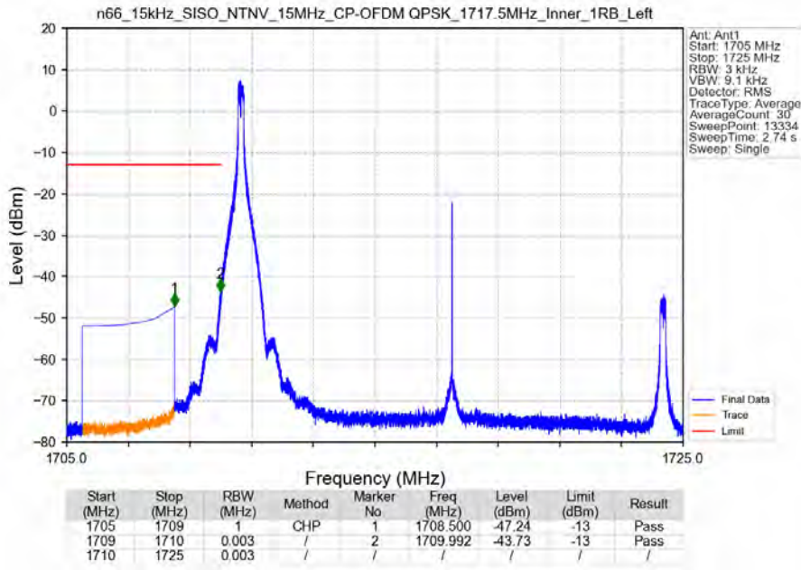
n66_15kHz_SISO_NTNV_15MHz_CP-OFDM QPSK_1717.5MHz_Inner_1RB_Left
