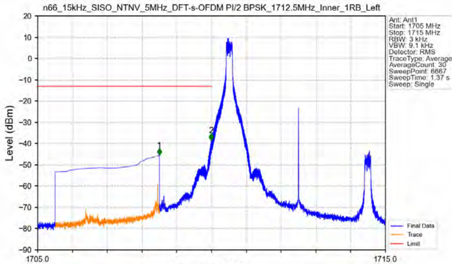
n66_15kHz_SISO_NTNV_5MHz_DFT-s-OFDM PI/2 BPSK_1712.5MHz_Inner_1RB_Left
