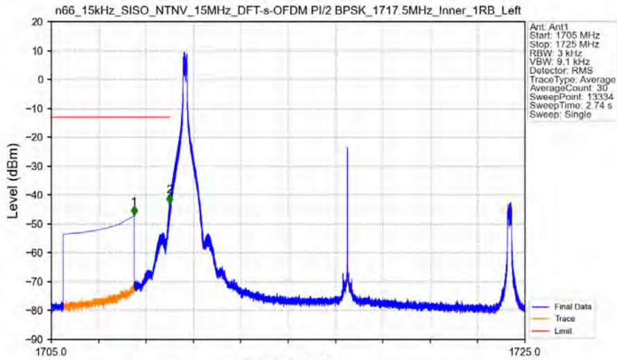
n66_15kHz_SISO_NTNV_15MHz_DFT-s-OFDM PI/2 BPSK_1717.5MHz_Inner_1RB_Left
