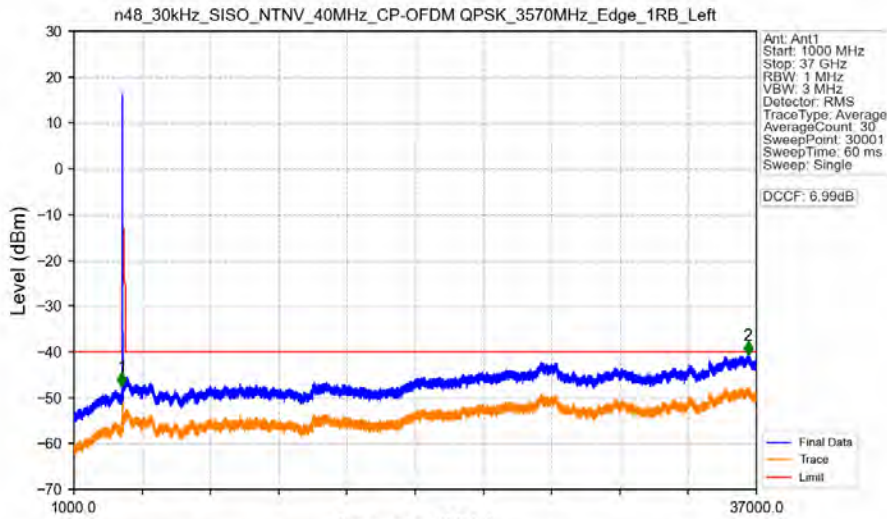
n48_30kHz_SISO_NTNV_40MHz_CP-OFDM QPSK_3570MHz_Edge_1RB_Left
