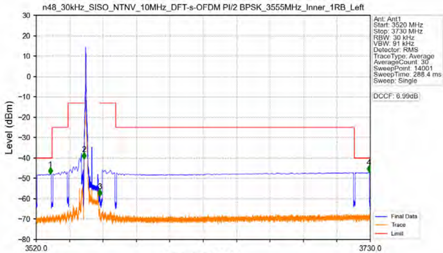
n48_30kHz_SISO_NTNV_10MHz_DFT-s-OFDM PI/2 BPSK_3555MHz_Inner_1RB_Left
