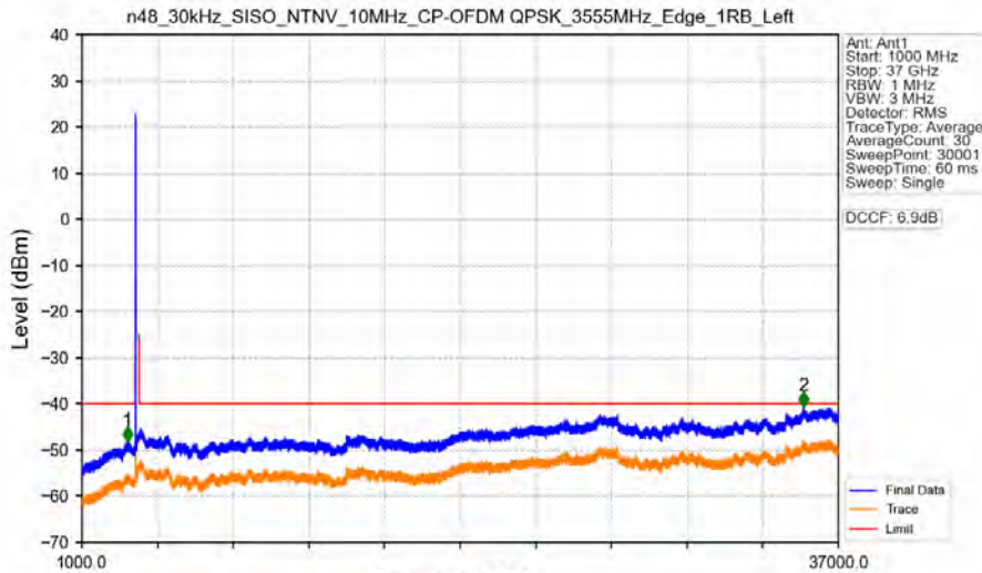
n48_30kHz_SISO_NTNV_10MHz_CP-OFDM QPSK_3555MHz_Edge_1RB_Left
