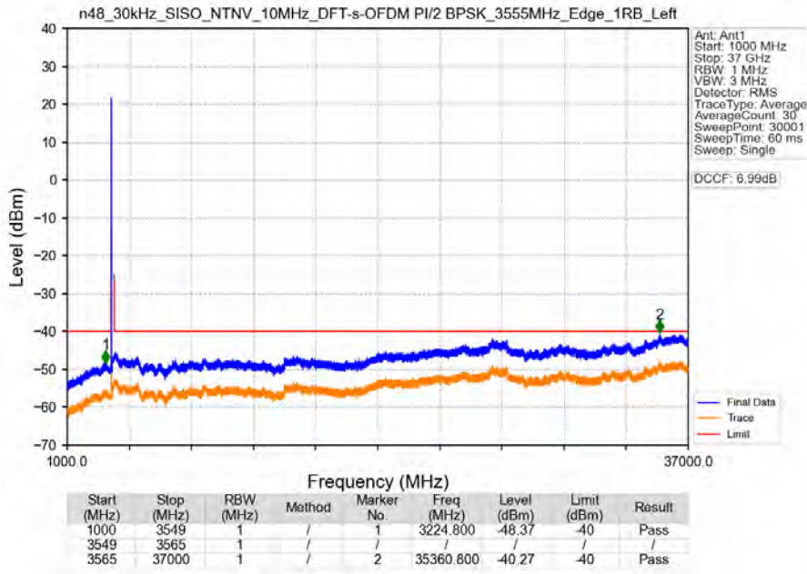
n48_30kHz_SISO_NTNV_10MHz_DFT-s-OFDM PI/2 BPSK_3555MHz_Edge_1RB_Left
