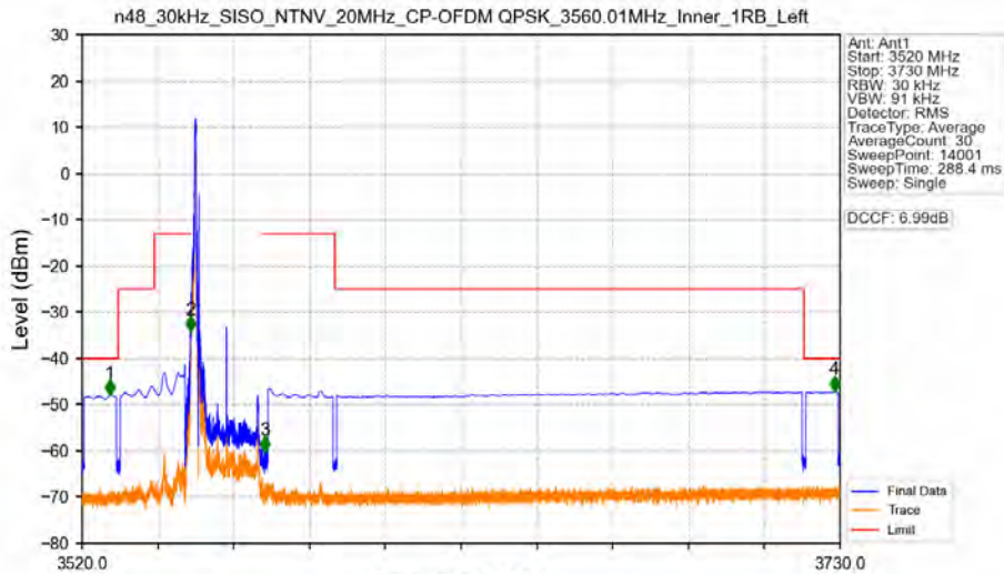
n48_30kHz_SISO_NTNV_20MHz_CP-OFDM QPSK_3560.01MHz_Inner_1RB_Left
