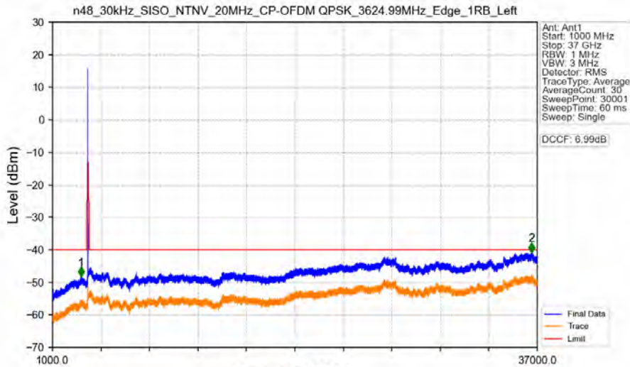
n48_30kHz_SISO_NTNV_20MHz_CP-OFDM QPSK_3624.99MHz_Edge_1RB_Left
