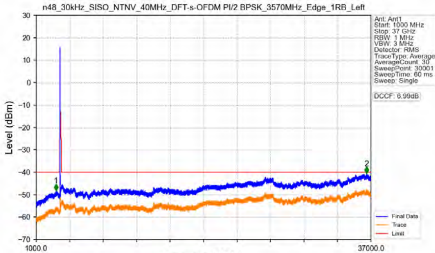
n48_30kHz_SISO_NTNV_40MHz_DFT-s-OFDM PI/2 BPSK_3570MHz_Edge_1RB_Left
