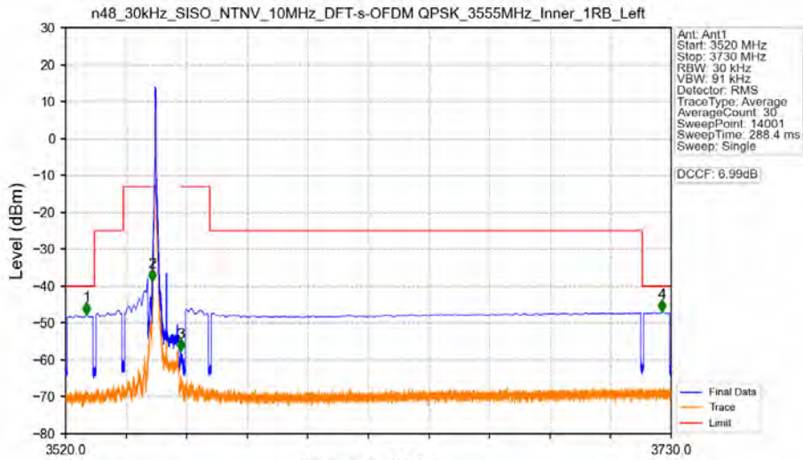
n48_30kHz_SISO_NTNV_10MHz_DFT-s-OFDM QPSK_3555MHz_Inner_1RB_Left
