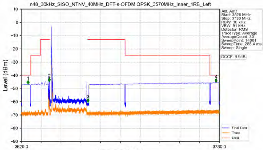
n48_30kHz_SISO_NTNV_40MHz_DFT-s-OFDM QPSK_3570MHz_Inner_1RB_Left
