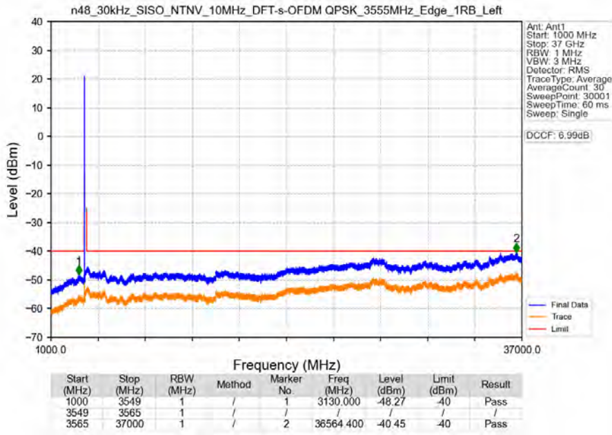
n48_30kHz_SISO_NTNV_10MHz_DFT-s-OFDM QPSK_3555MHz_Edge_1RB_Left
