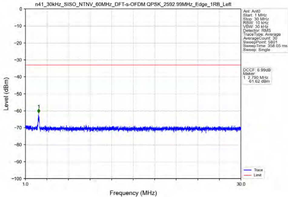
n41_30kHz_SISO_NTNV_60MHz_DFT-s-OFDM QPSK_2592.99MHz_Edge_1RB_Left
