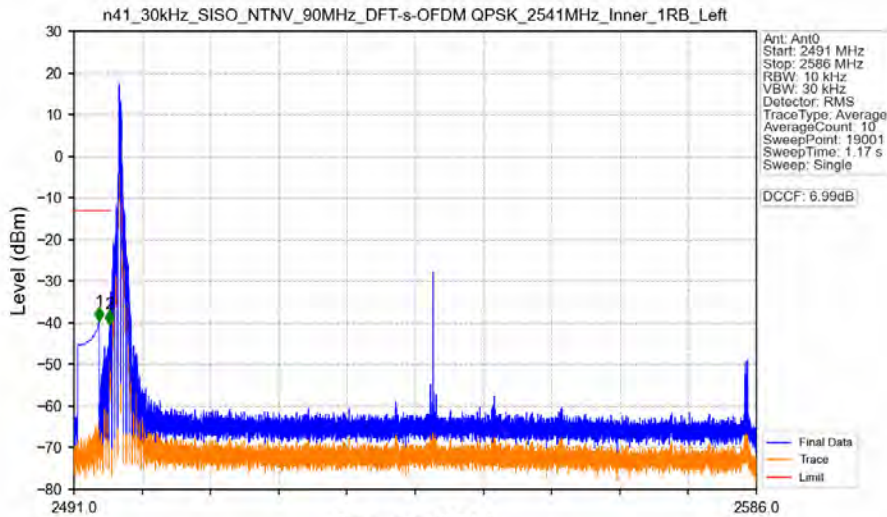
n41_30kHz_SISO_NTNV_90MHz_DFT-s-OFDM QPSK_2541MHz_Inner_1RB_Left
