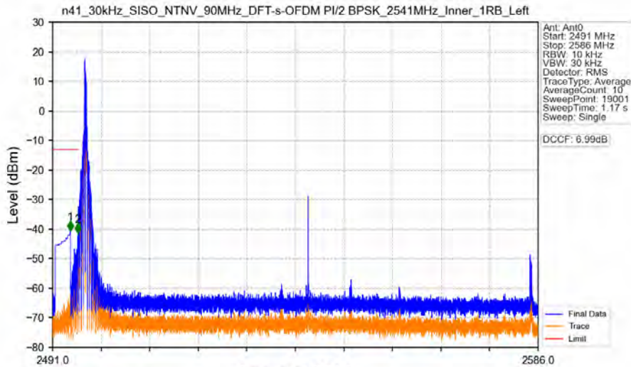
n41_30kHz_SISO_NTNV_90MHz_DFT-s-OFDM PI/2 BPSK_2541MHz_Inner_1RB_Left
