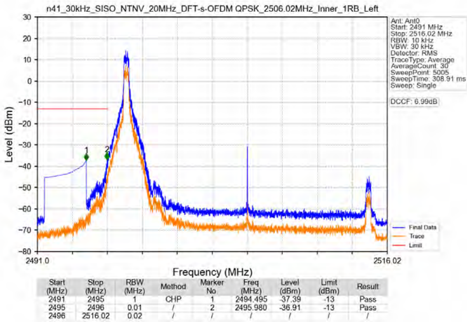
n41_30kHz_SISO_NTNV_20MHz_DFT-s-OFDM QPSK_2506.02MHz_Inner_1RB_Left
