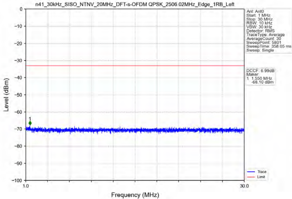
n41_30kHz_SISO_NTNV_20MHz_DFT-s-OFDM QPSK_2506.02MHz_Edge_1RB_Left
