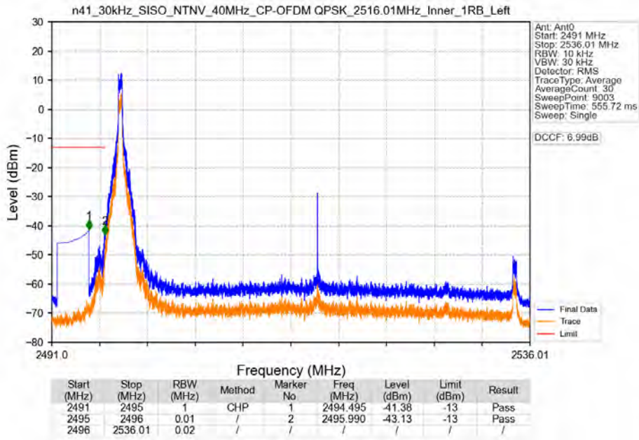
n41_30kHz_SISO_NTNV_40MHz_CP-OFDM QPSK_2516.01MHz_Inner_1RB_Left
