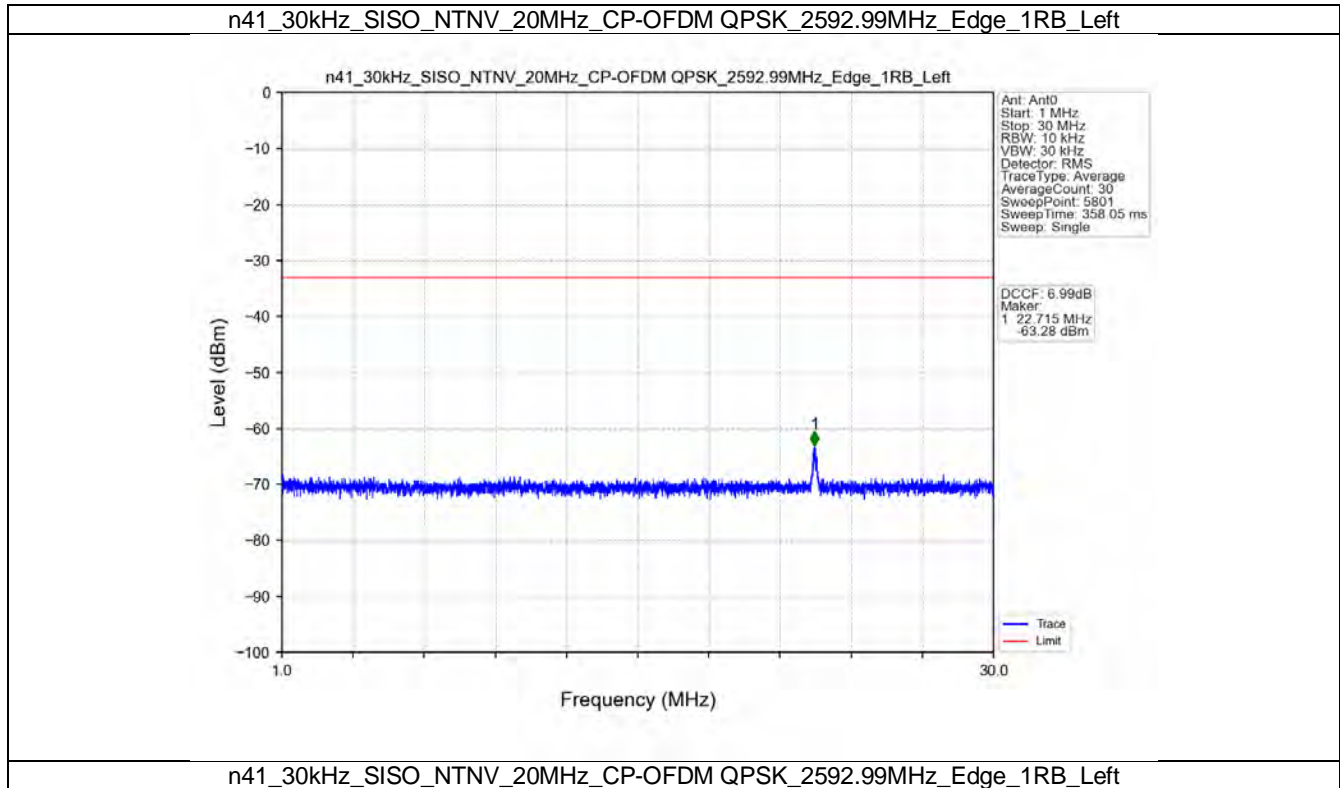
n41_30kHz_SISO_NTNV_20MHz_CP-OFDM QPSK_2592.99MHz_Edge_1RB_Left
