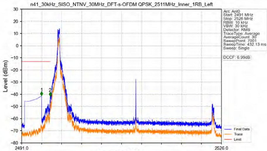
n41_30kHz_SISO_NTNV_30MHz_DFT-s-OFDM_QPSK_2511MHz_Inner_1RB_Left
