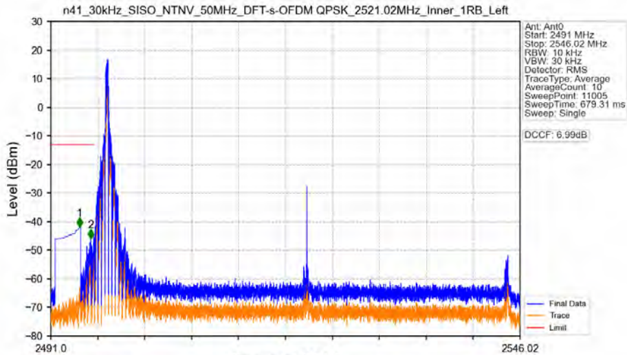
n41_30kHz_SISO_NTNV_50MHz_DFT-s-OFDM QPSK_2521.02MHz_Inner_1RB_Left
