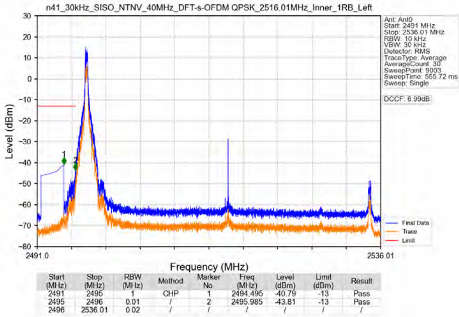
n41_30kHz_SISO_NTNV_40MHz_DFT-s-OFDM QPSK_2516.01MHz_Inner_1RB_Left
