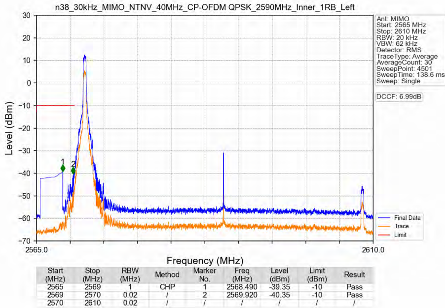
n38_30kHz_MIMO_NTNV_40MHz_CP-OFDM QPSK_2590MHz_Inner_1RB_Left
