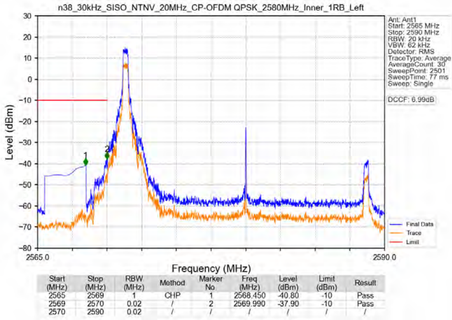
n38_30kHz_SISO_NTNV_20MHz_CP-OFDM QPSK_2580MHz_Inner_1RB_Left
