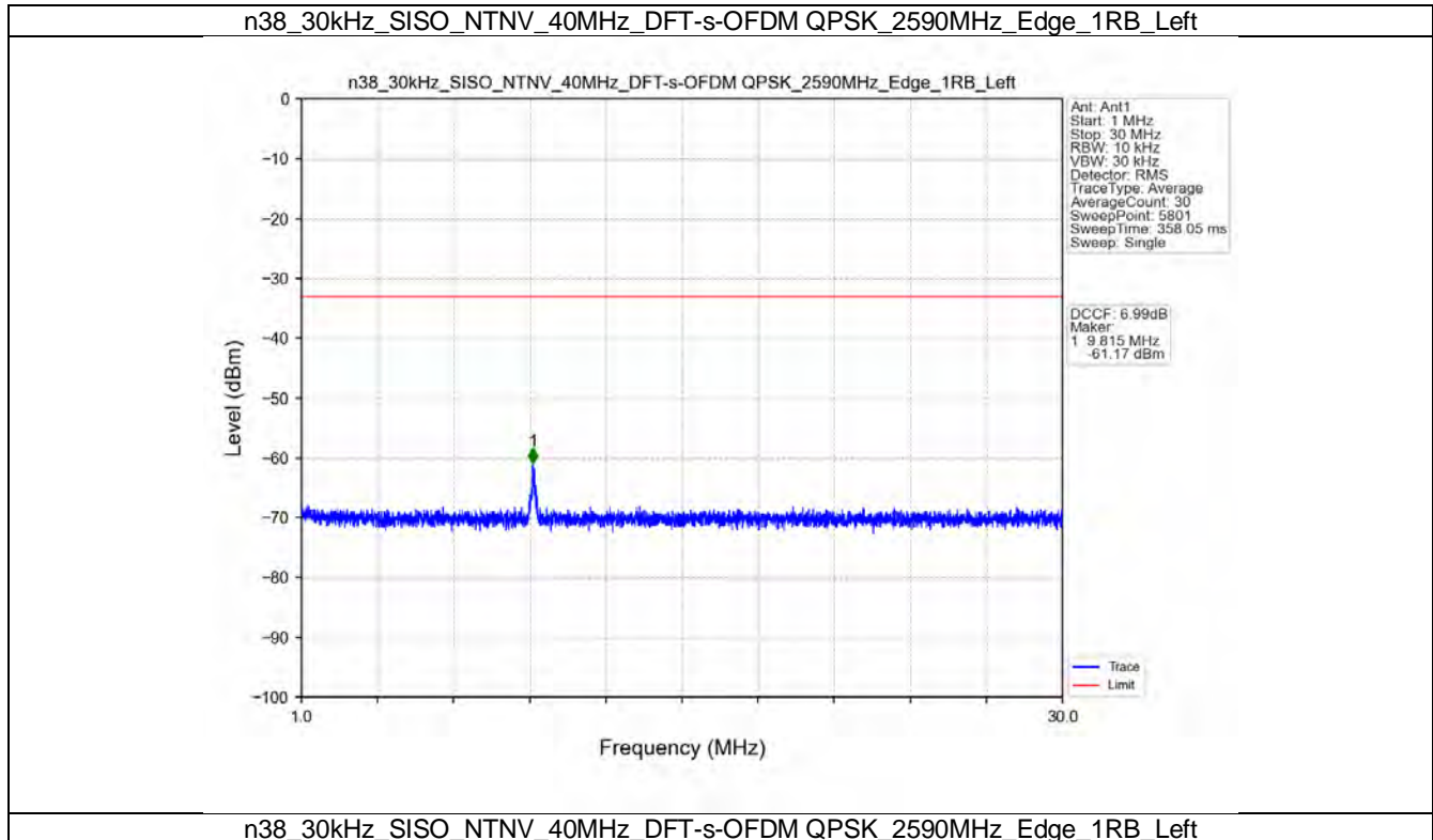
n38_30kHz_SISO_NTNV_40MHz_DFT-s-OFDM_QPSK_2590MHz_Edge_1RB_Left
