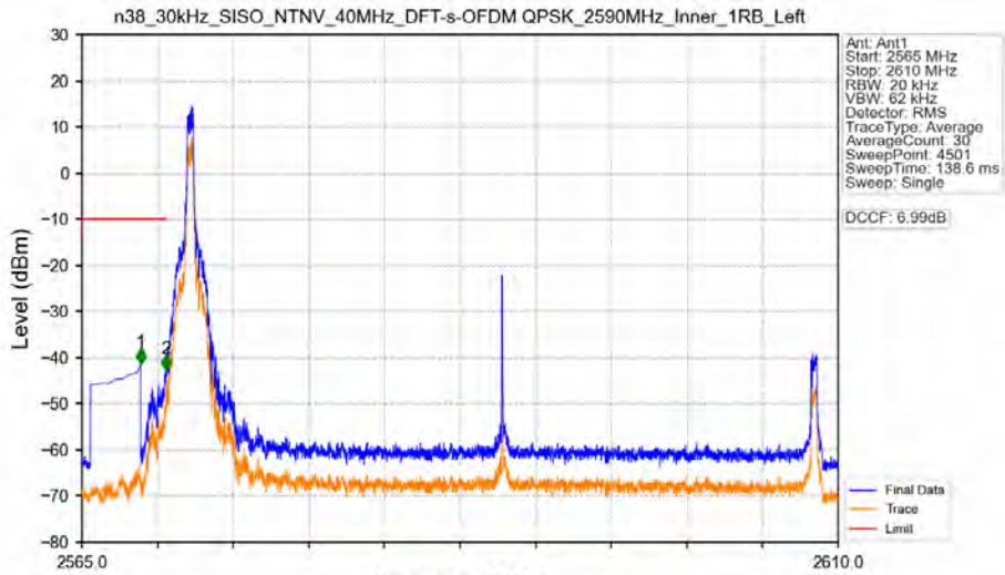
n38_30kHz_SISO_NTNV_40MHz_DFT-s-OFDM_QPSK_2590MHz_Inner_1RB_Left
