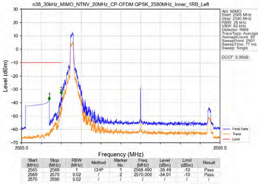
n38_30kHz_MIMO_NTNV_20MHz_CP-OFDM QPSK_2580MHz_Inner_1RB_Left
