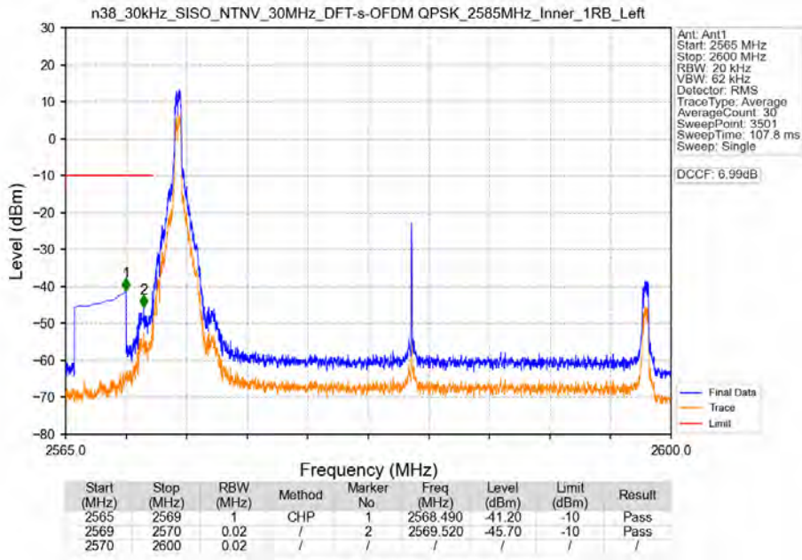
n38_30kHz_SISO_NTNV_30MHz_DFT-s-OFDM_QPSK_2585MHz_Inner_1RB_Left
