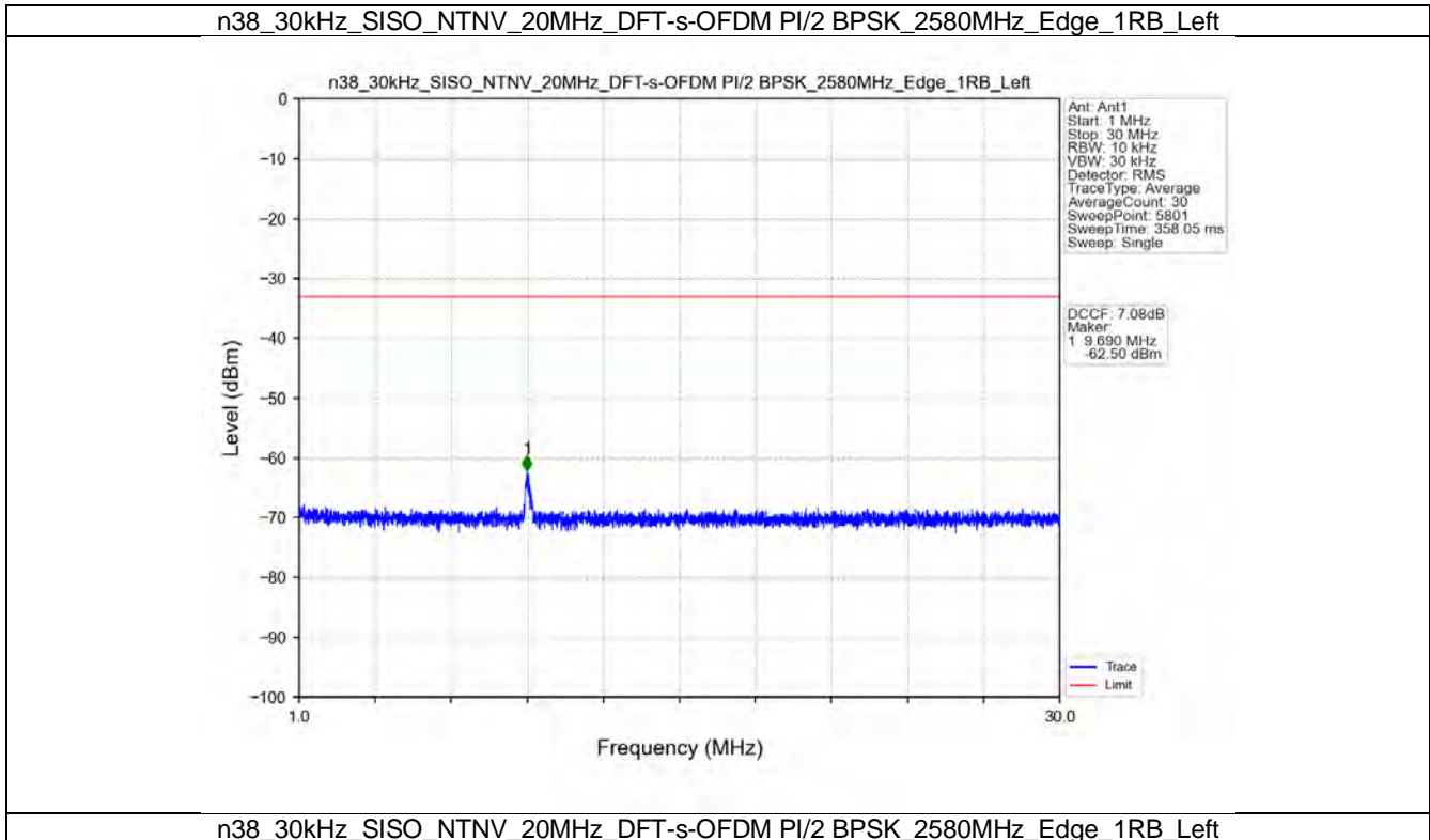
n38_30kHz_SISO_NTNV_20MHz_DFT-s-OFDM_PI/2_BPSK_2580MHz_Edge_1RB_Left
