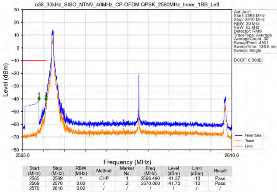
n38_30kHz_SISO_NTNV_40MHz_CP-OFDM QPSK_2590MHz_Inner_1RB_Left
