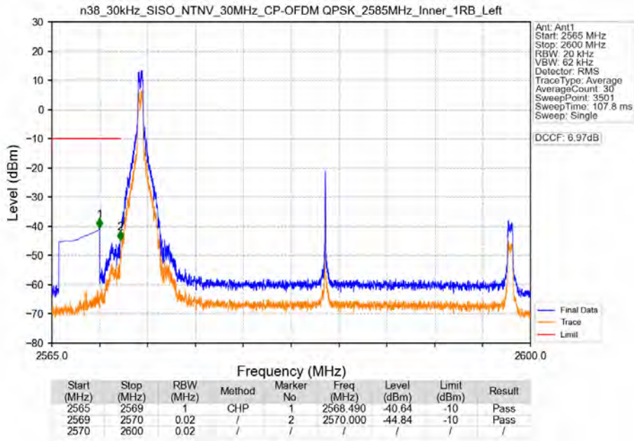
n38_30kHz_SISO_NTNV_30MHz_CP-OFDM QPSK_2585MHz_Inner_1RB_Left
