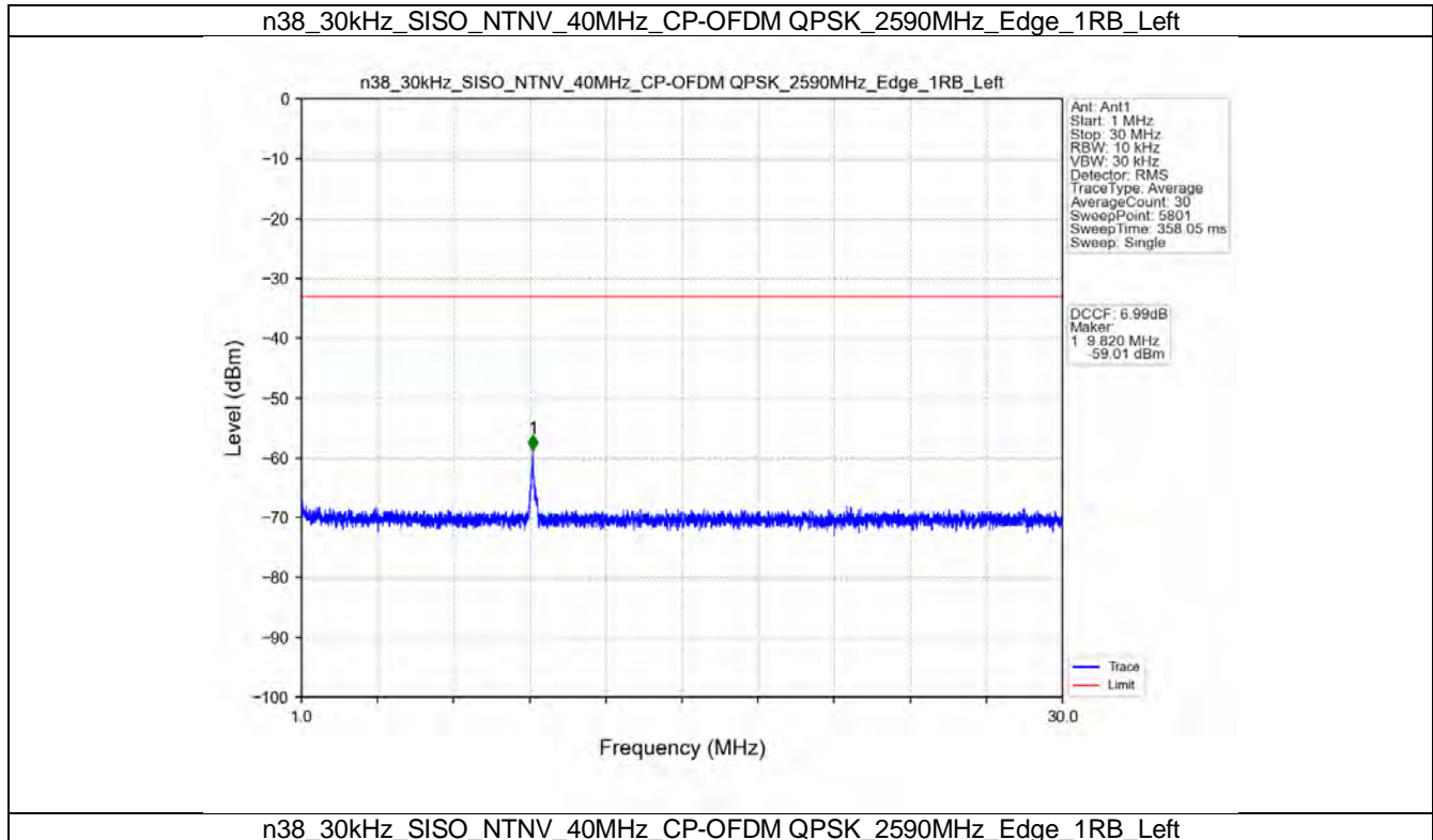
n38_30kHz_SISO_NTNV_40MHz_CP-OFDM QPSK_2590MHz_Edge_1RB_Left
