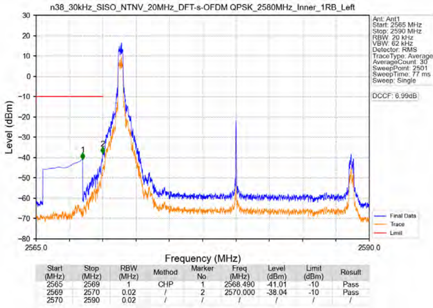
n38_30kHz_SISO_NTNV_20MHz_DFT-s-OFDM QPSK_2580MHz_Inner_1RB_Left
